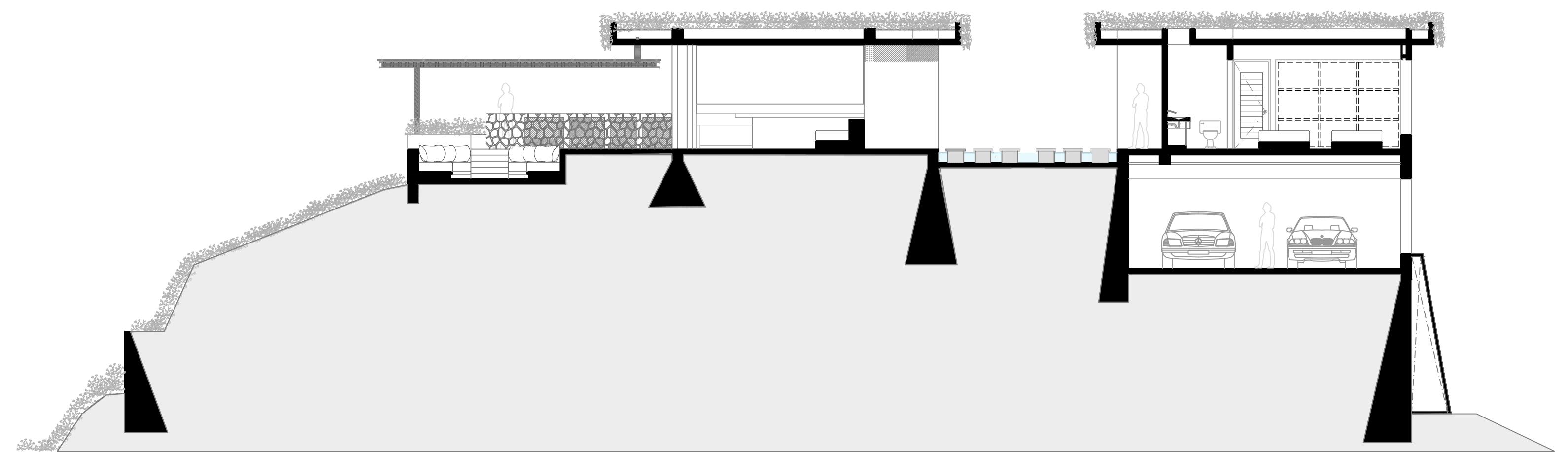
CORTE XX1
