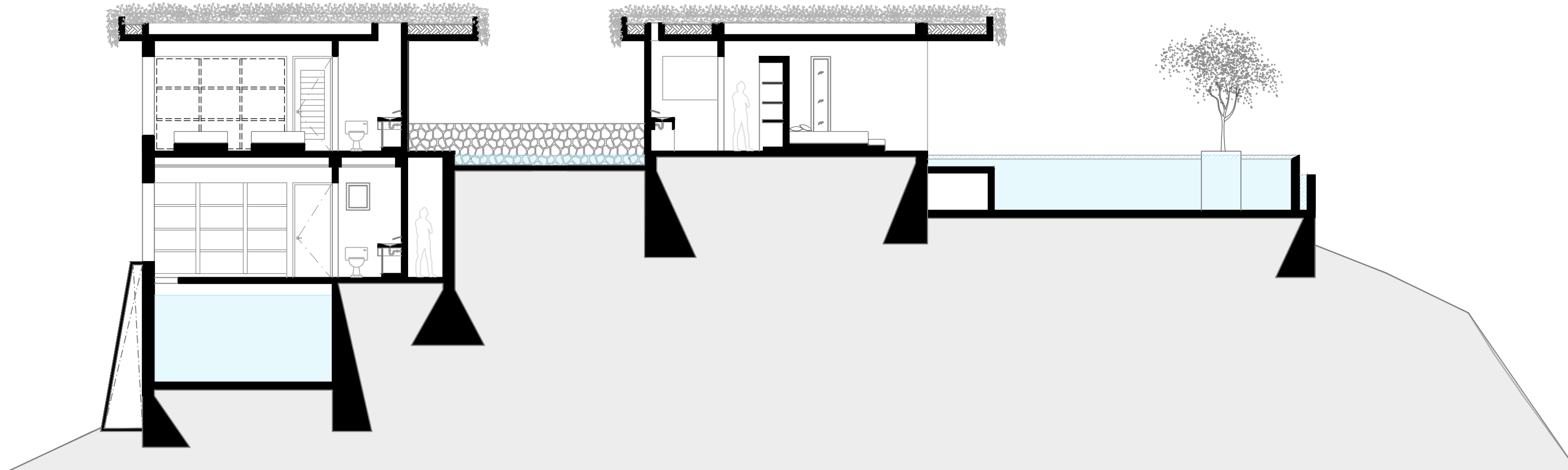
CORTE ZZ1
