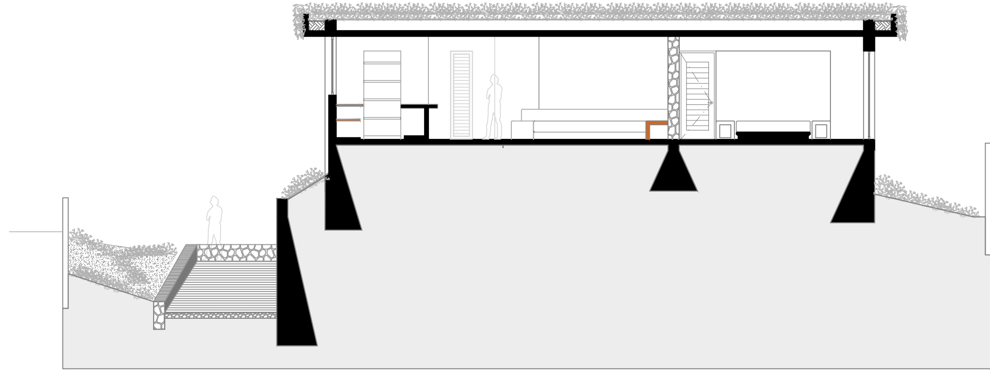
CORTE SS1
