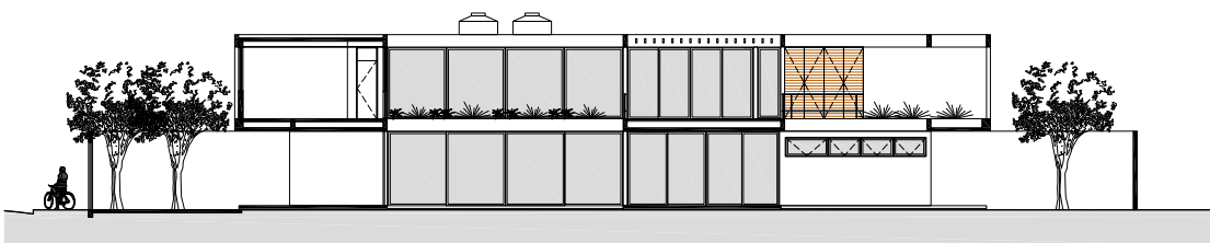
0 1 2 5 CORTE BB' SECTION BB'
