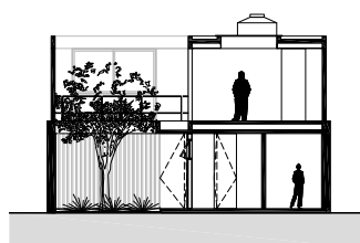
0 1 2 5 CORTE EE' SECTION EE'
