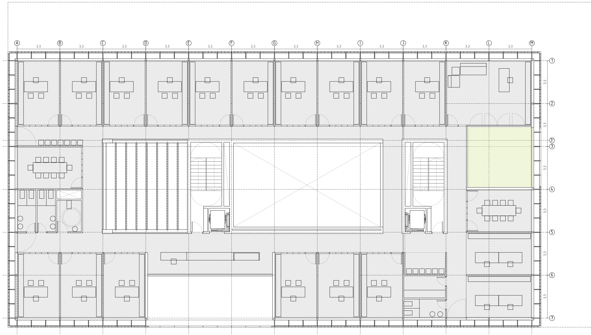
E 1:150 PLANTA SEGUNDA
