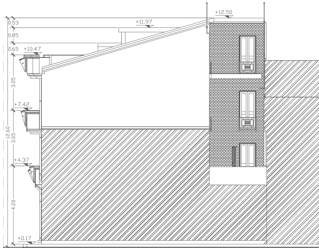
Prospetto Sud-Est
