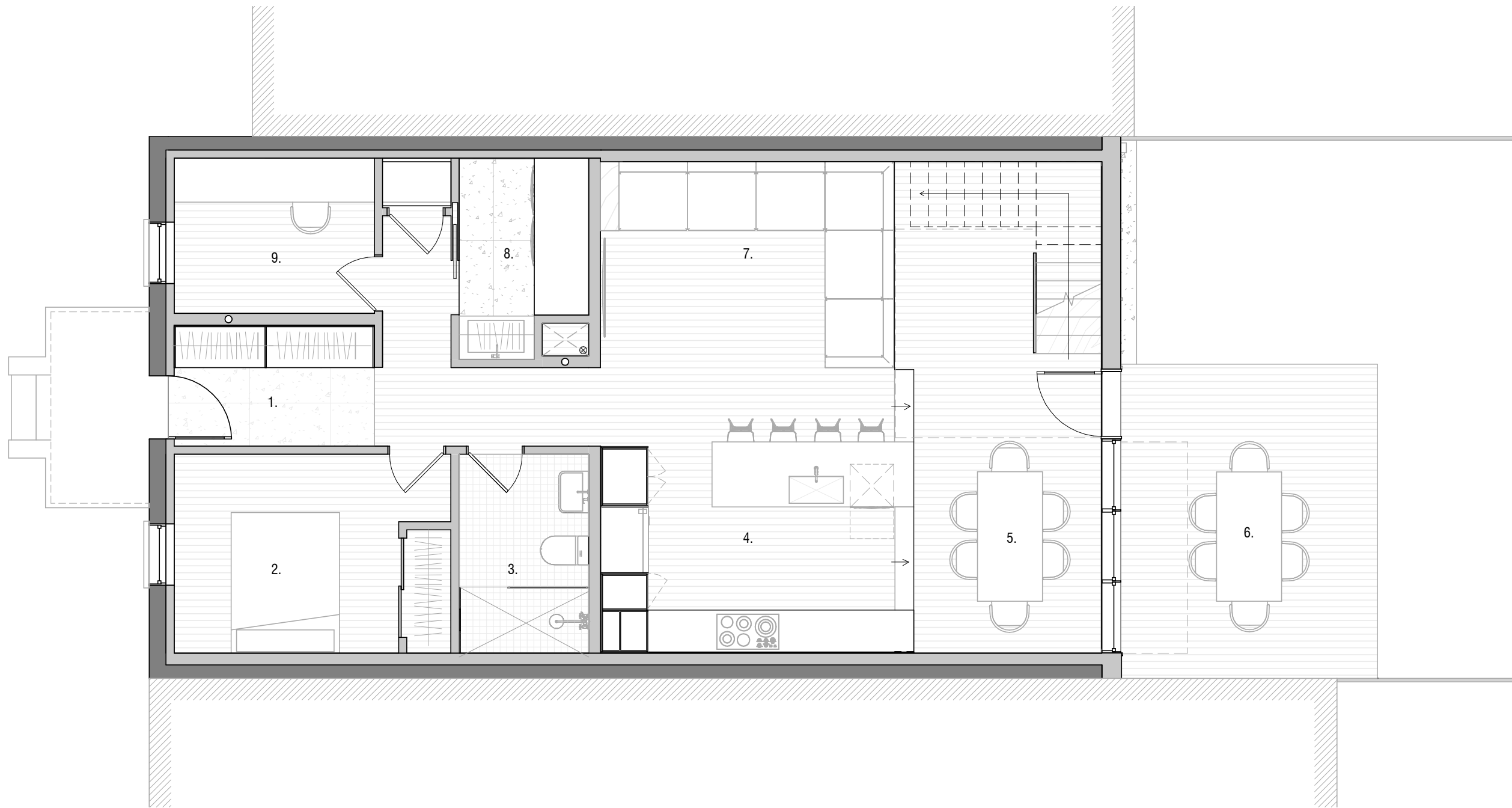
PLAN REZ-DE-CHAUSSÉE
