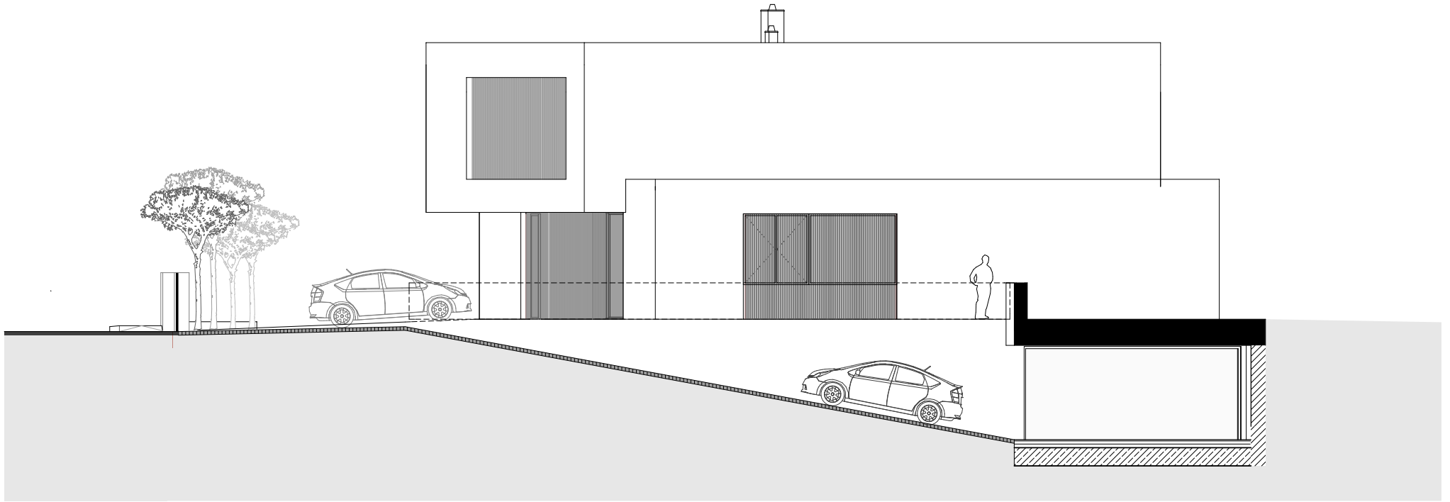
Ansicht Nord-West M 1:100
