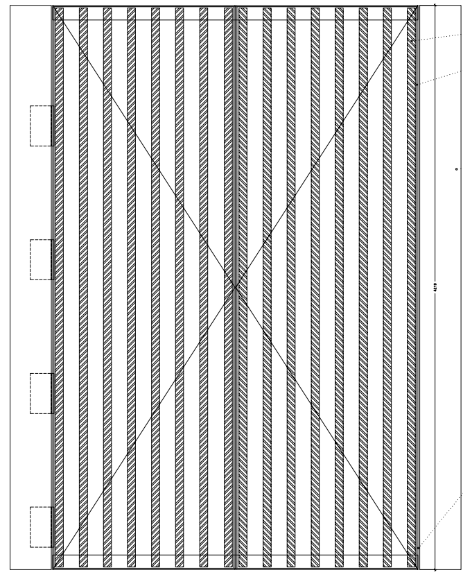
FACHADA TIPO4 PORTONES ABATIBLES, MARCO DE PASANANOS DE 100mm CON LAMAS DE MADERA PE 10x40cm A TORNJLLAS DETALLE 1/10 EN MM
