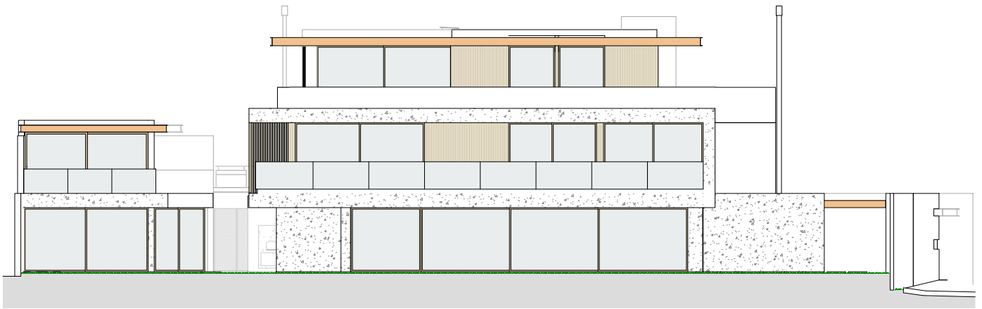
ELEVAÇÃO 2
