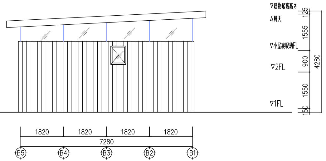
西側立面図
