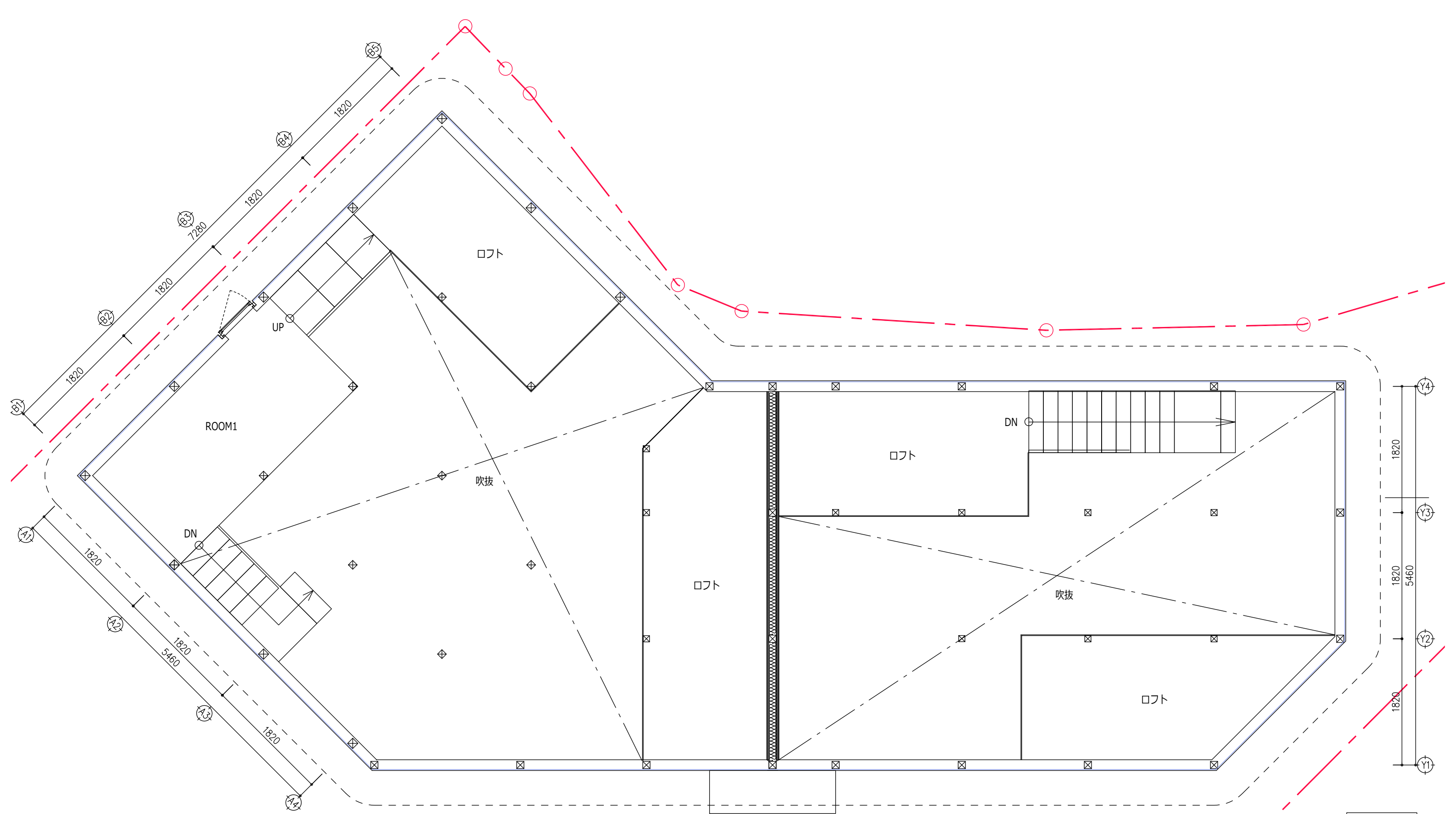
2階平面図
