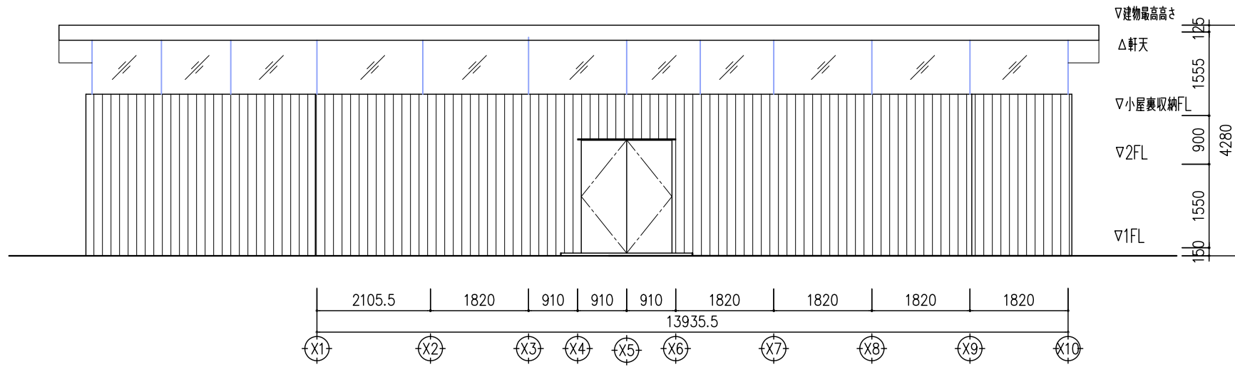
南側立面図
