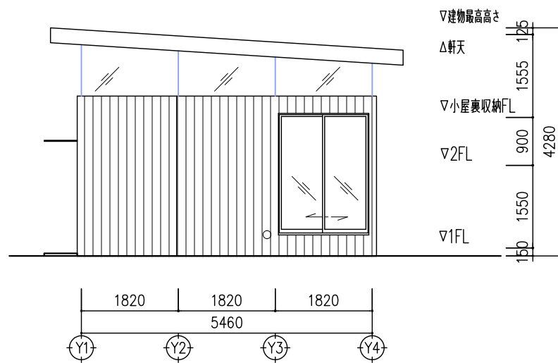
東側立面図
