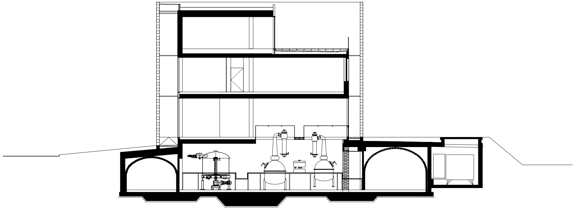
SCHNITT 1-1
