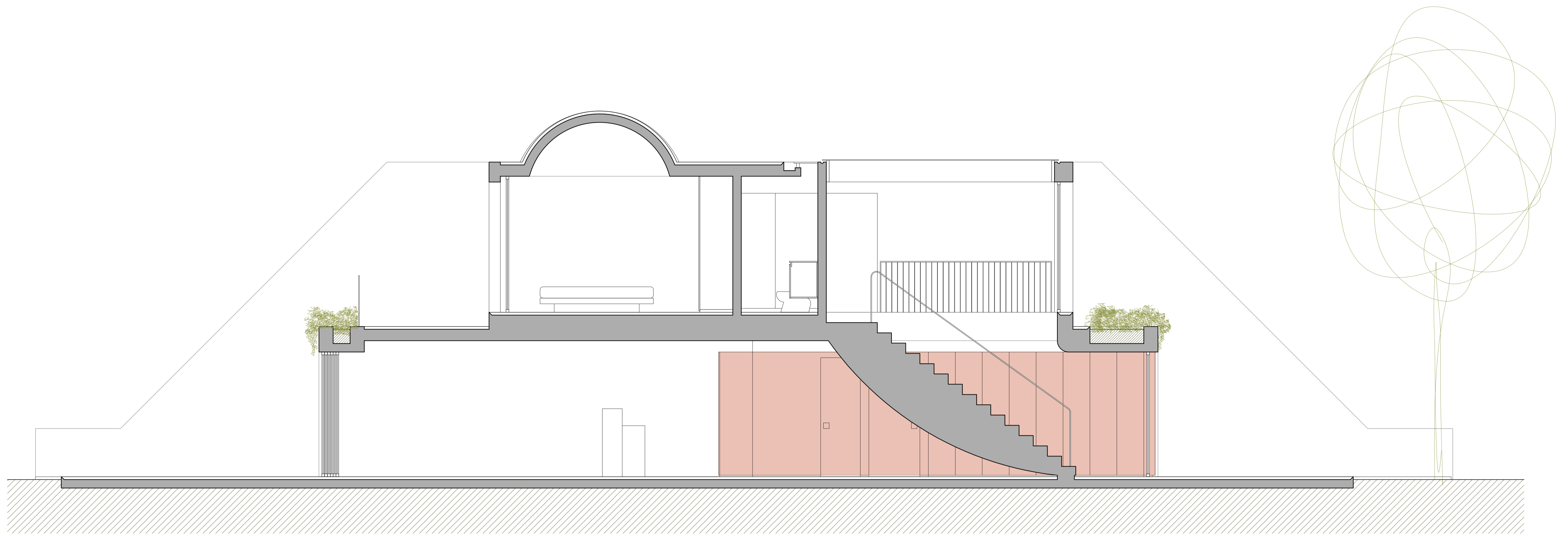
CORTE B
