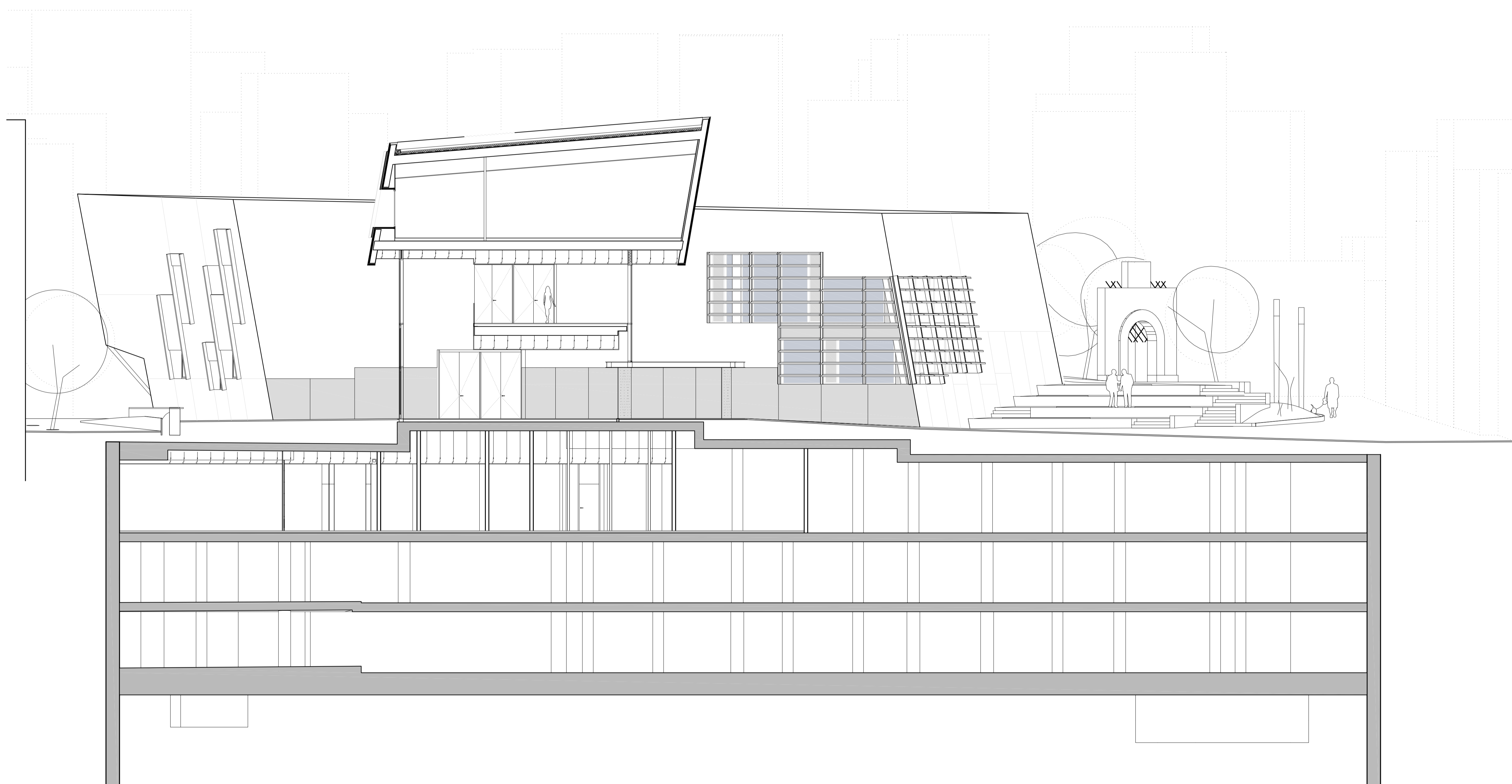
LONGITUDINAL SECTION 2
