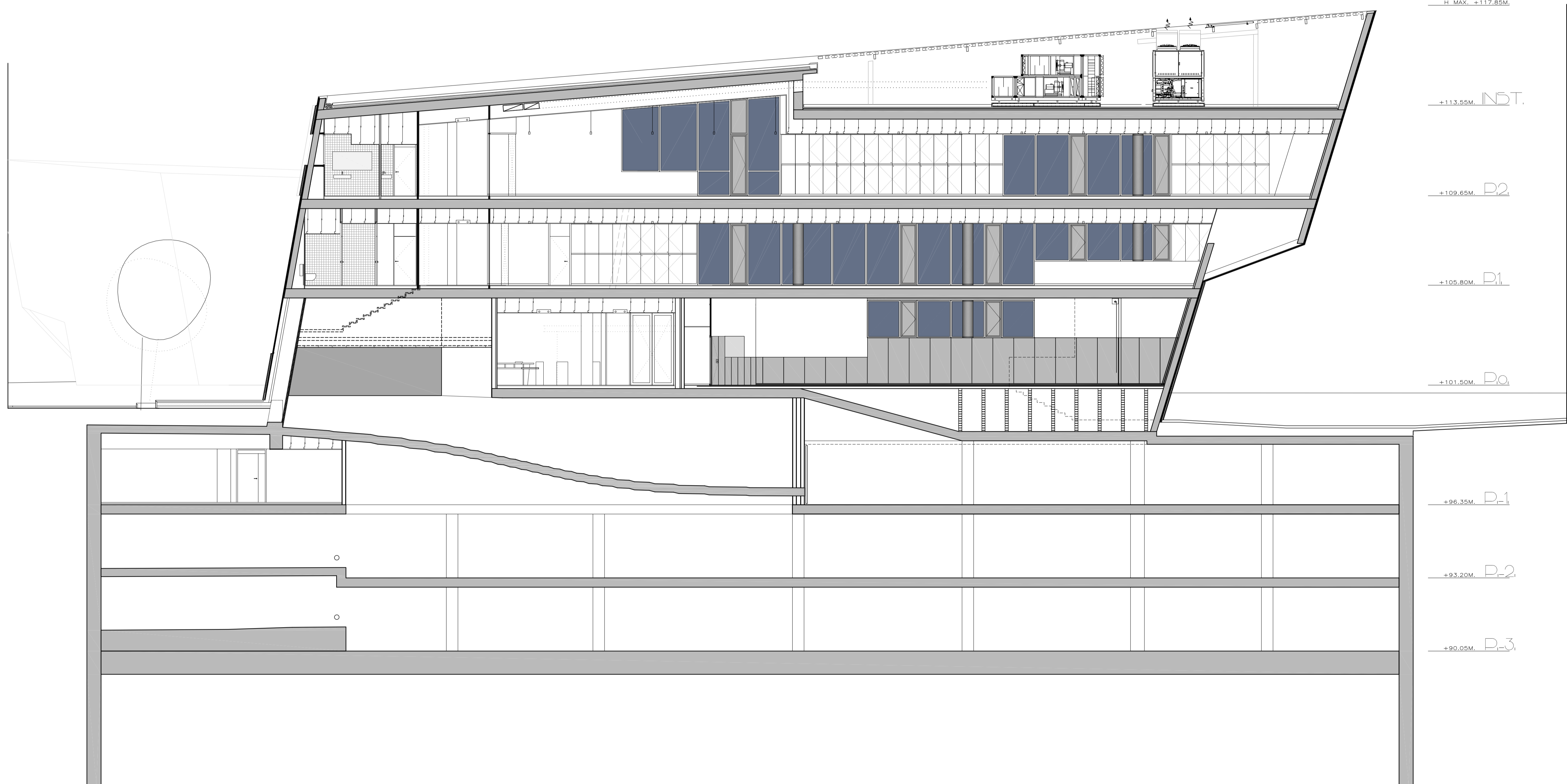
LONGITUDINAL SECTION 1
