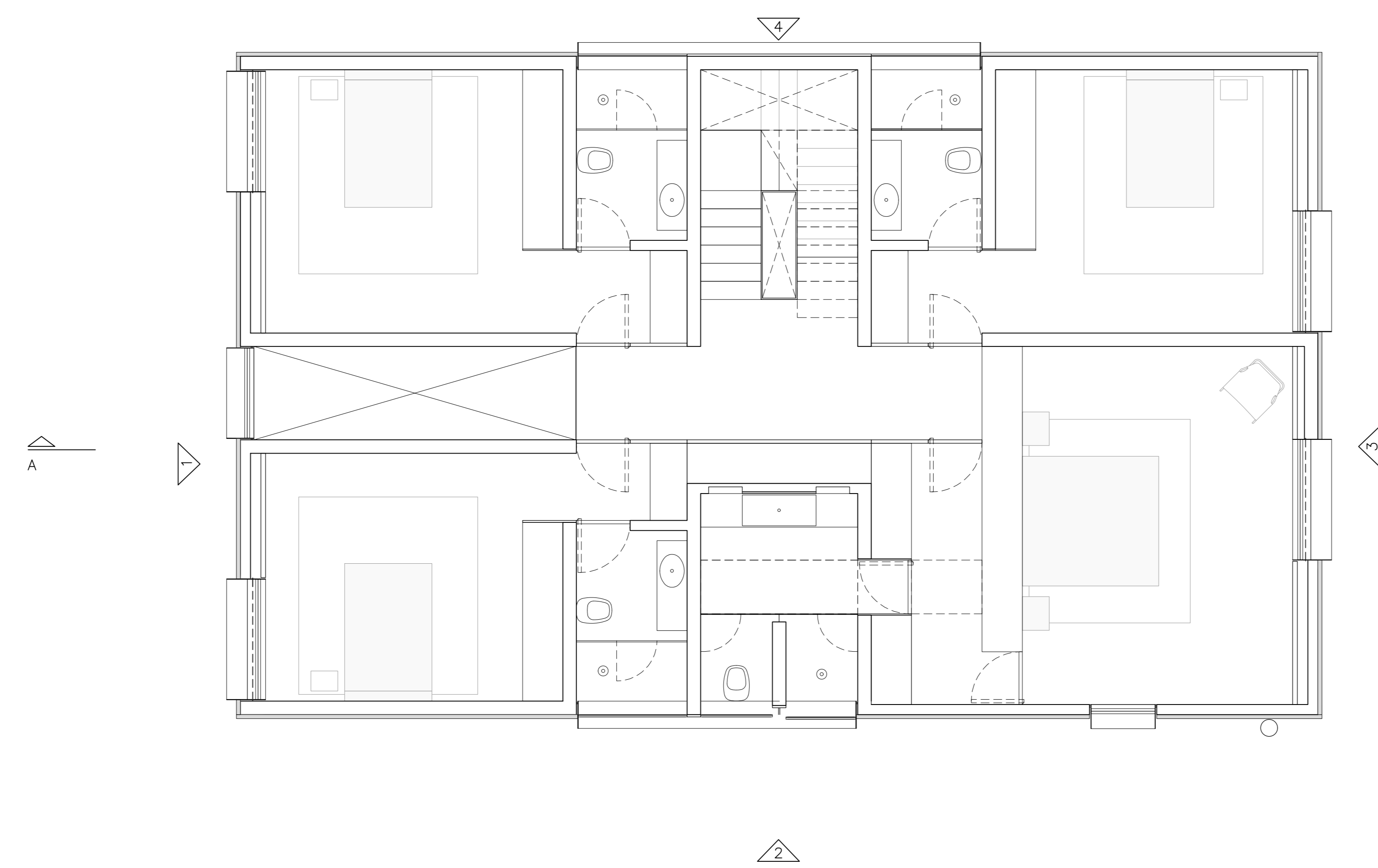
PLANTA - PAVIMENTO SUPERIOR
