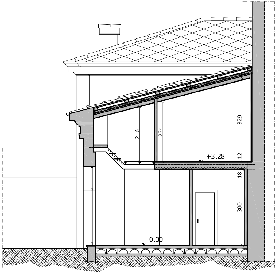
SEZIONE A-A'
