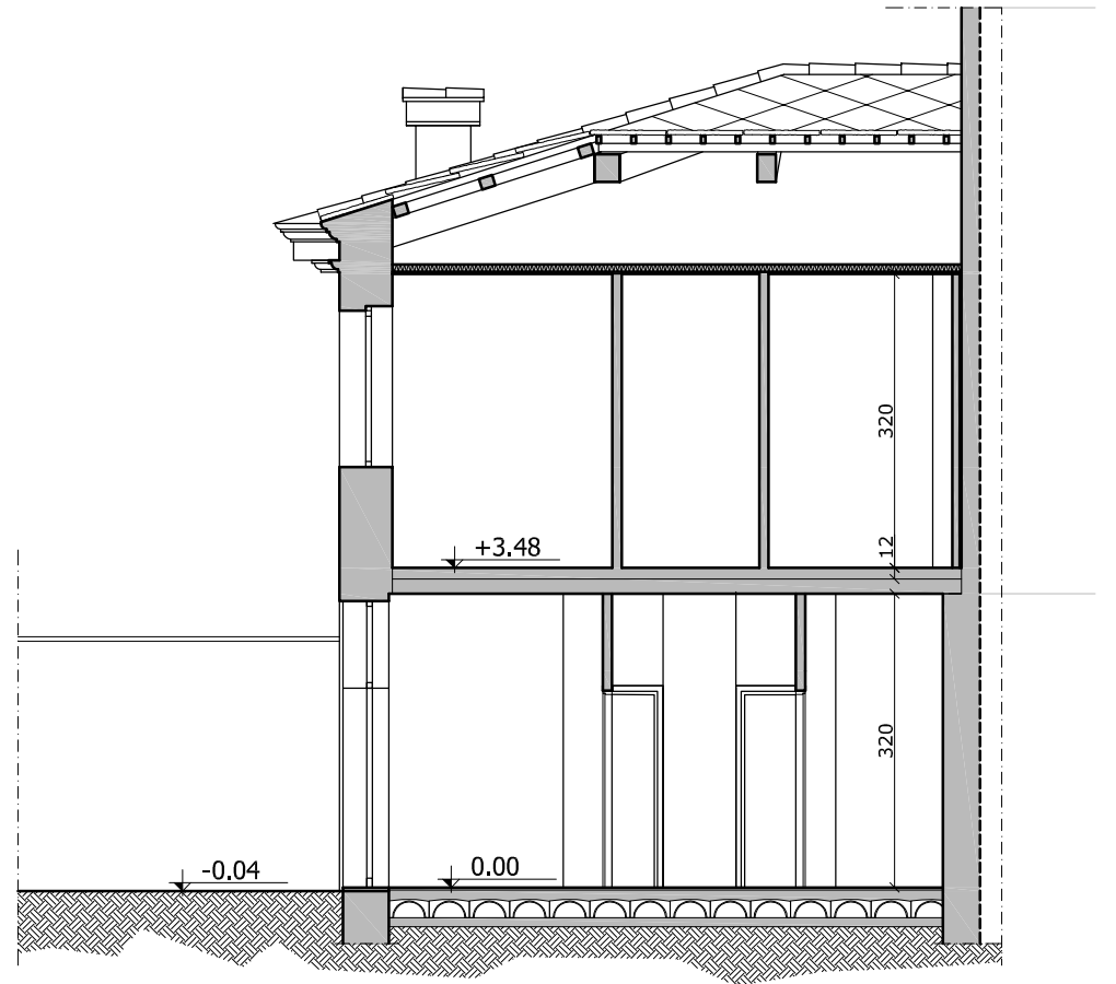
SEZIONE B-B'
