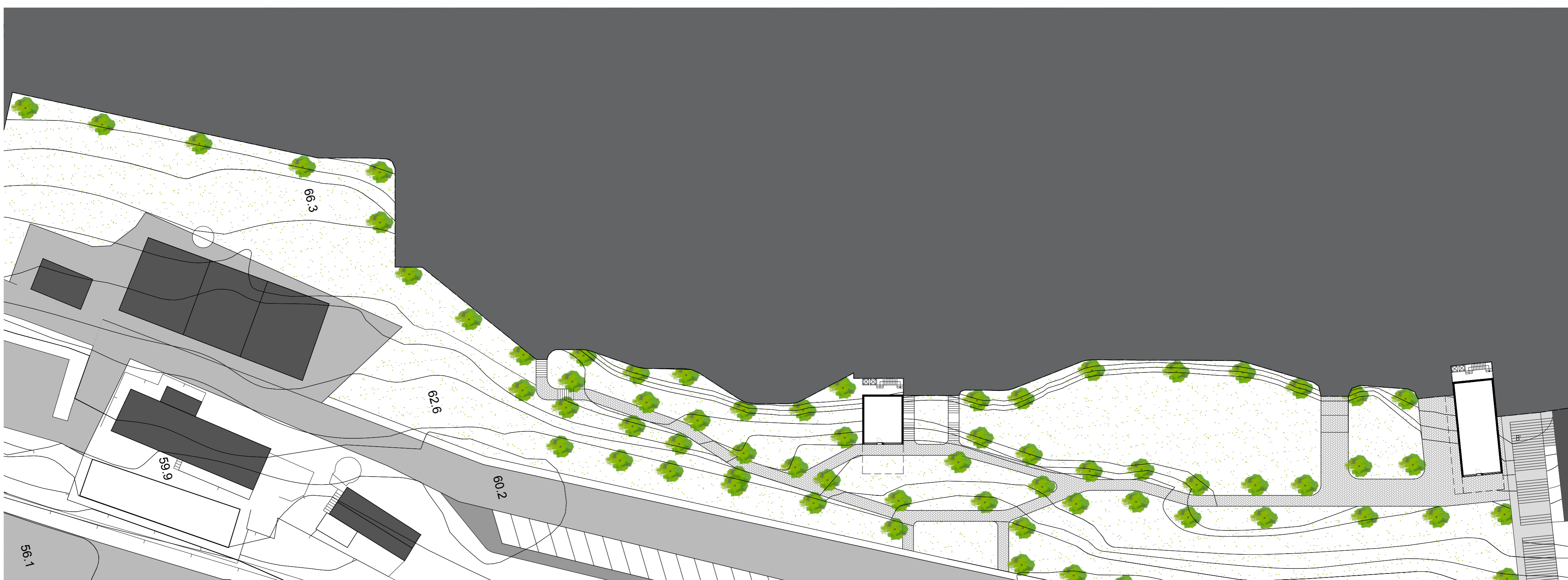
Planta à cota 68.2m Esc:1/500
