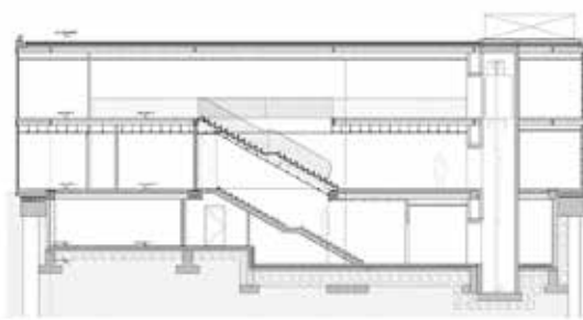
Sezione longitudinale
