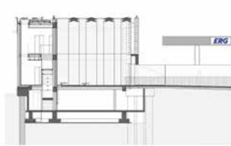
Sezione trasversale
