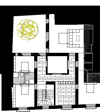
PLANTA 1ª. ESTADO REFORMADO.
