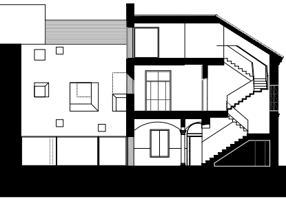
SECCIÓN E-E
