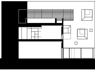
SECCIÓN D-D
