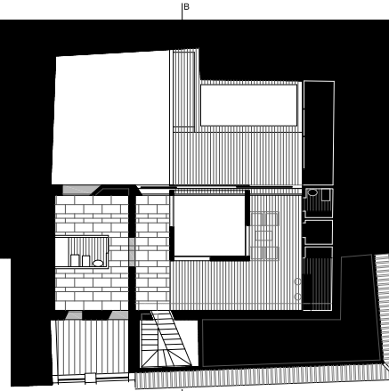
PLANTA 2ª. ESTADO REFORMADO.
