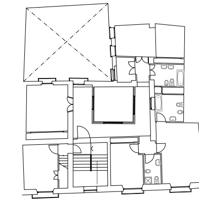
PLANTA 1ª. ESTADO PREVIO.
