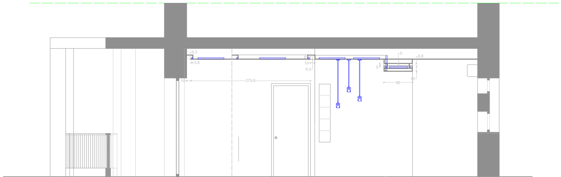
Sez A-A
