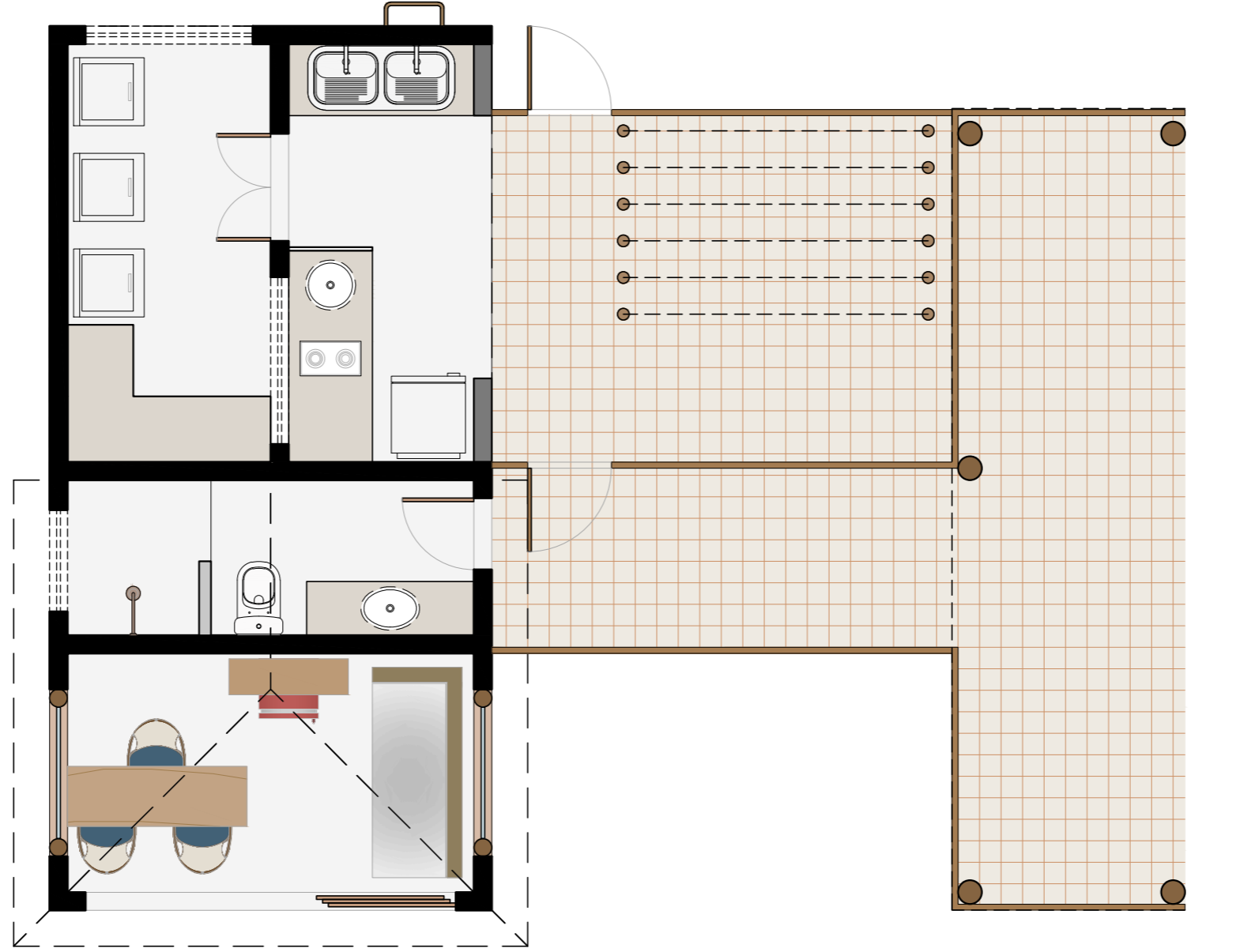
POUSADA HAYÔ | TÉRREO RECEPÇÃO / I.S. FUNCIONÁRIOS / LAVANDERIA | PLANTA LAYOUT
