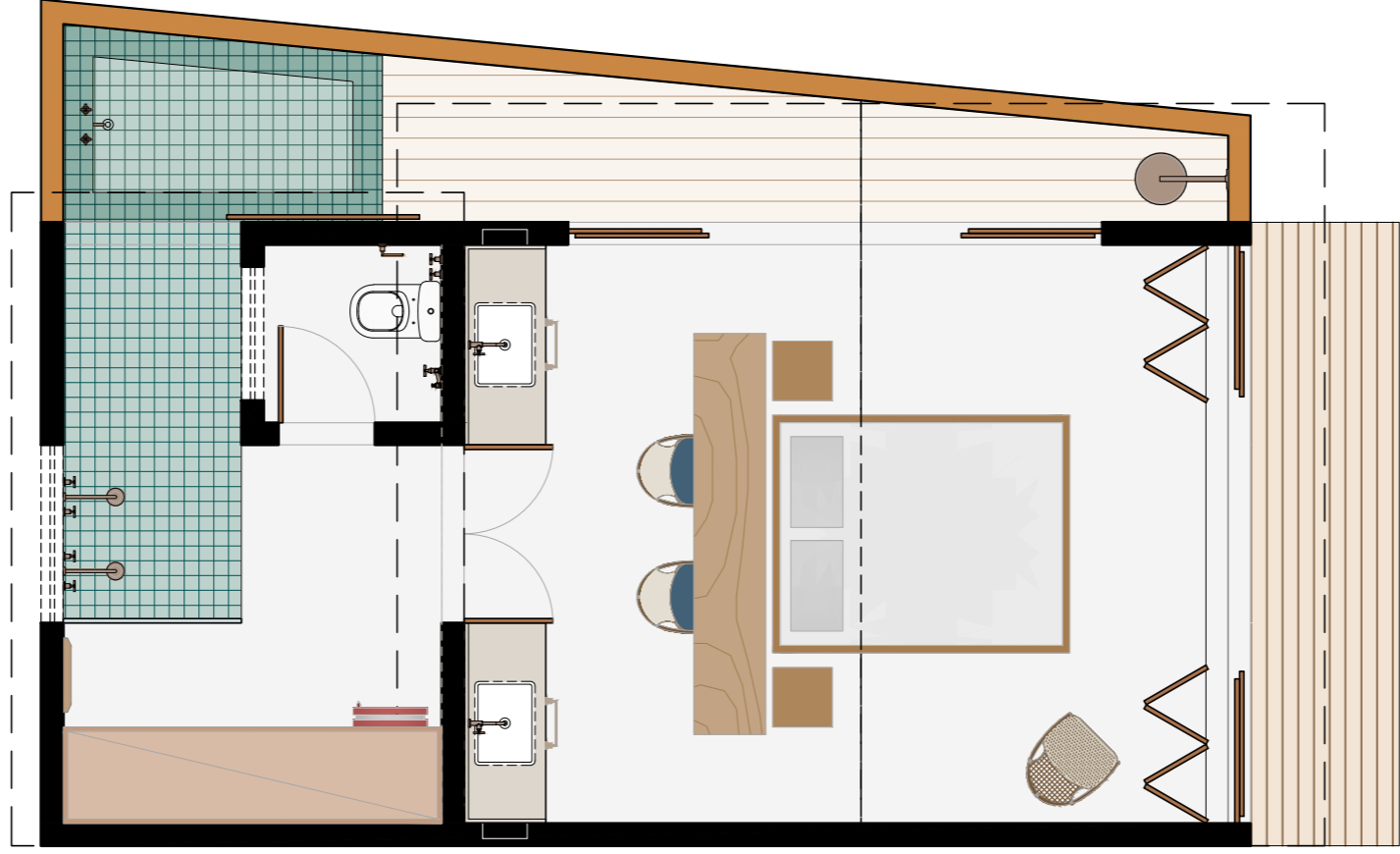
POUSADA HAYÔ | TÉRREO SUÍTE 3 | PLANTA LAYOUT
