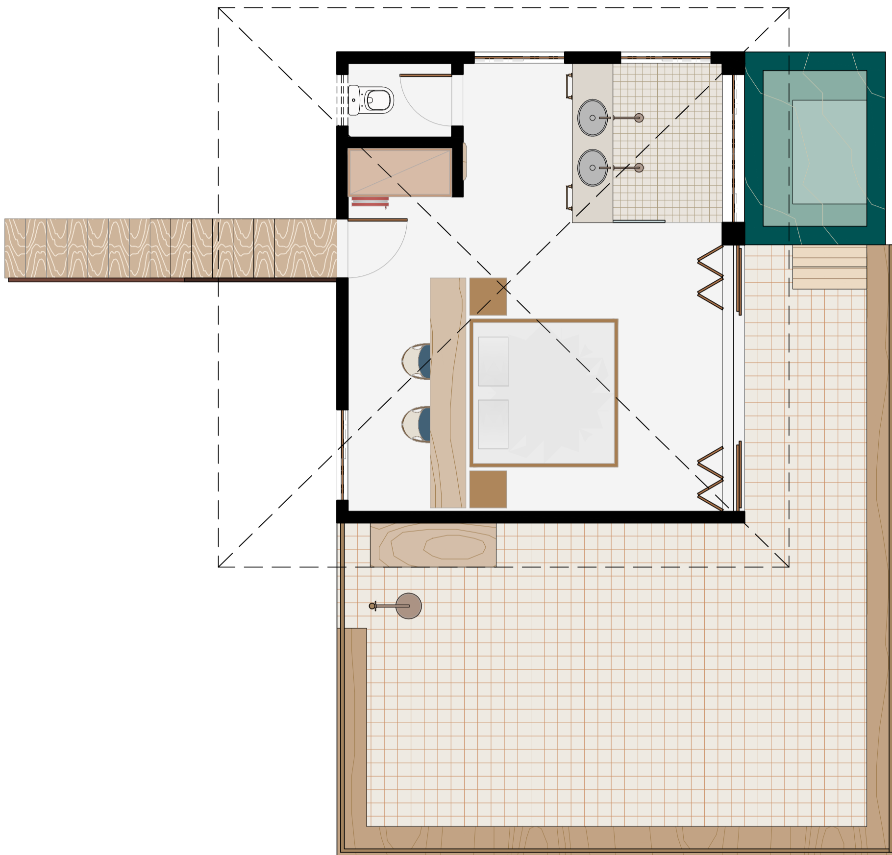
POUSADA HAYÔ | 2º PAVIMENTO SUÍTE 4 | PLANTA LAYOUT
