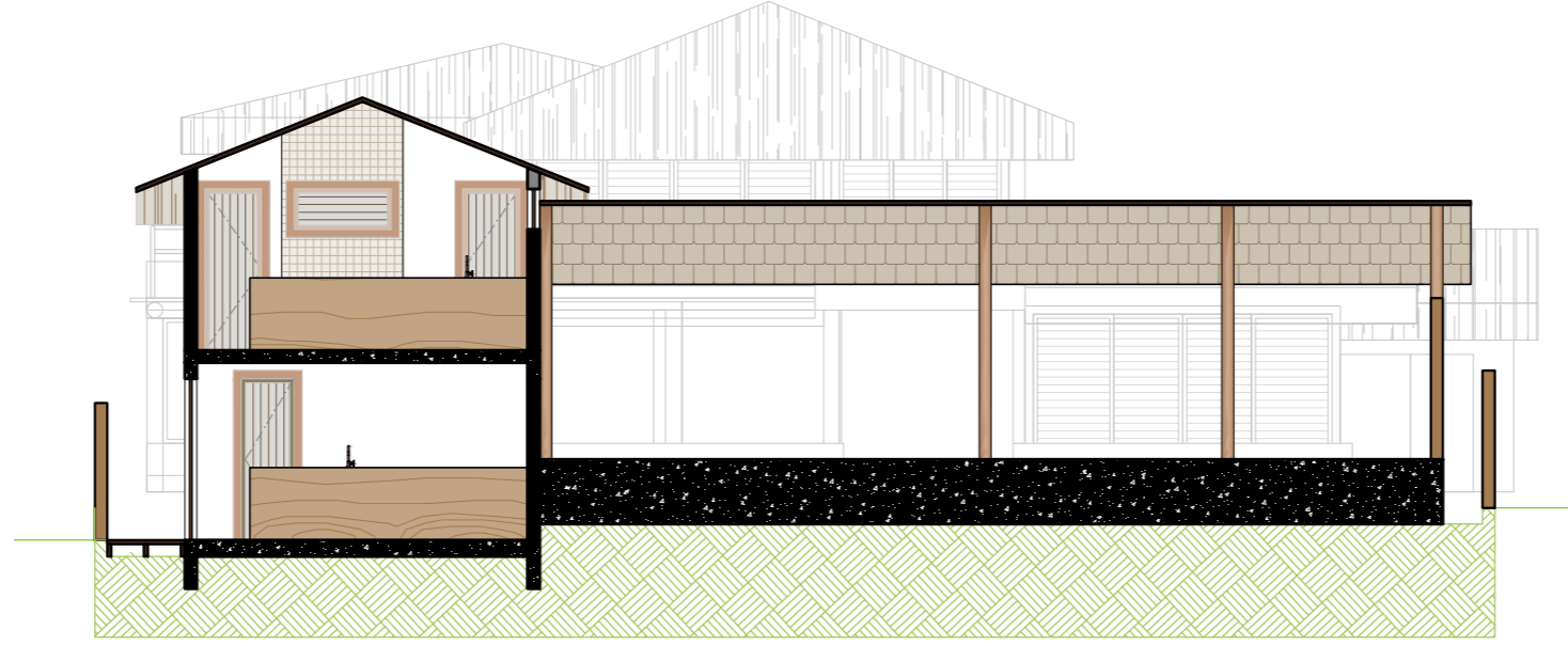
POUSADA HAYÔ CORTE E
