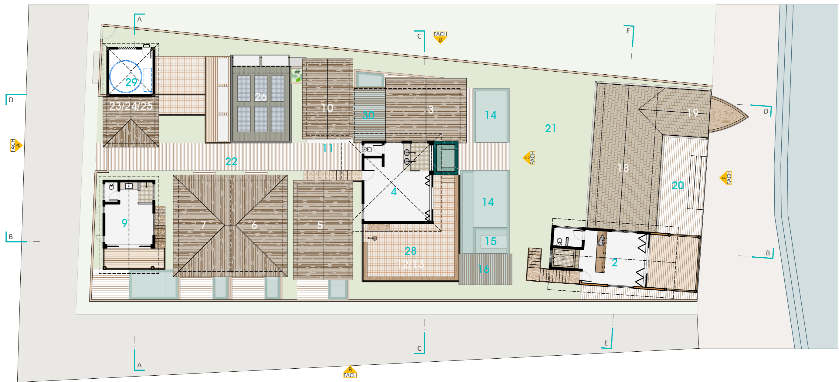
POUSADA HAYÔ PLANTA DE IMPLANTAÇÃO | 2º PAVIMENTO 0 0.5 1 2 5 10m N
