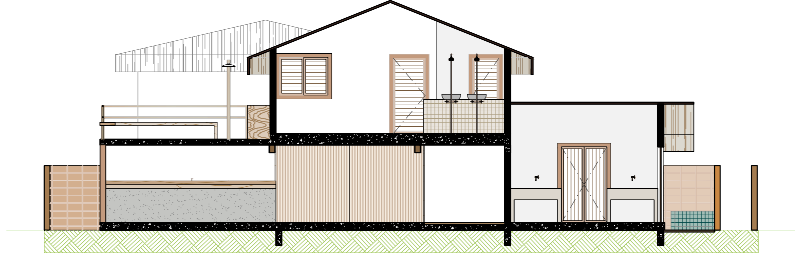
POUSADA HAYÓ CORTE C
