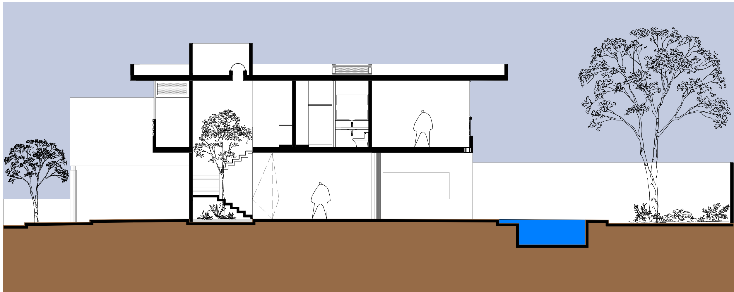
CORTE B-B'
