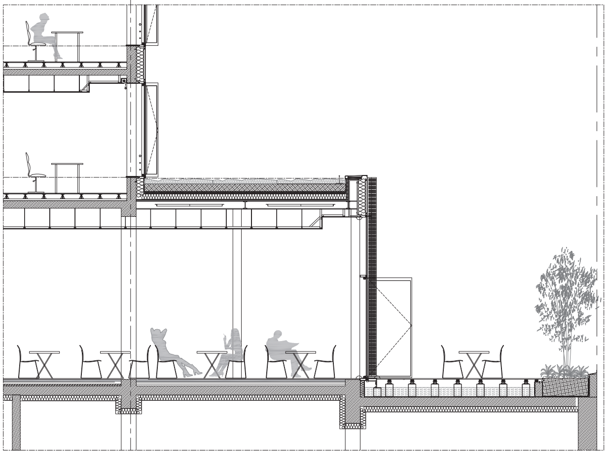
COUPE A-A
