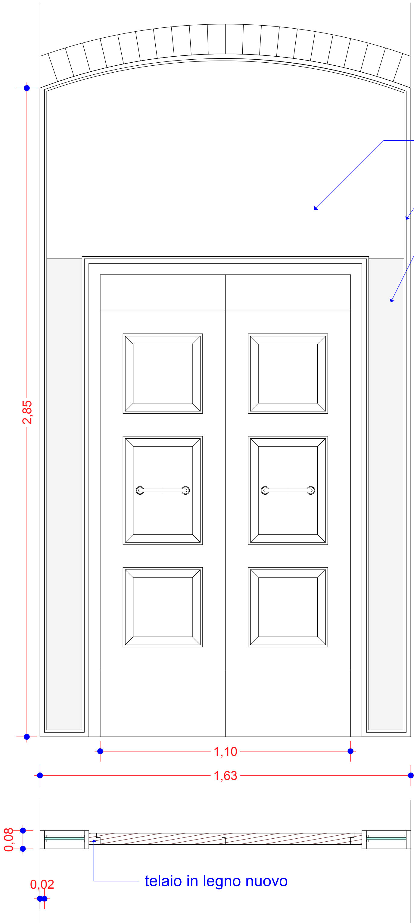
PORTA INGRESSO RECUPERATA prospetto e pianta rapp: 1/10
