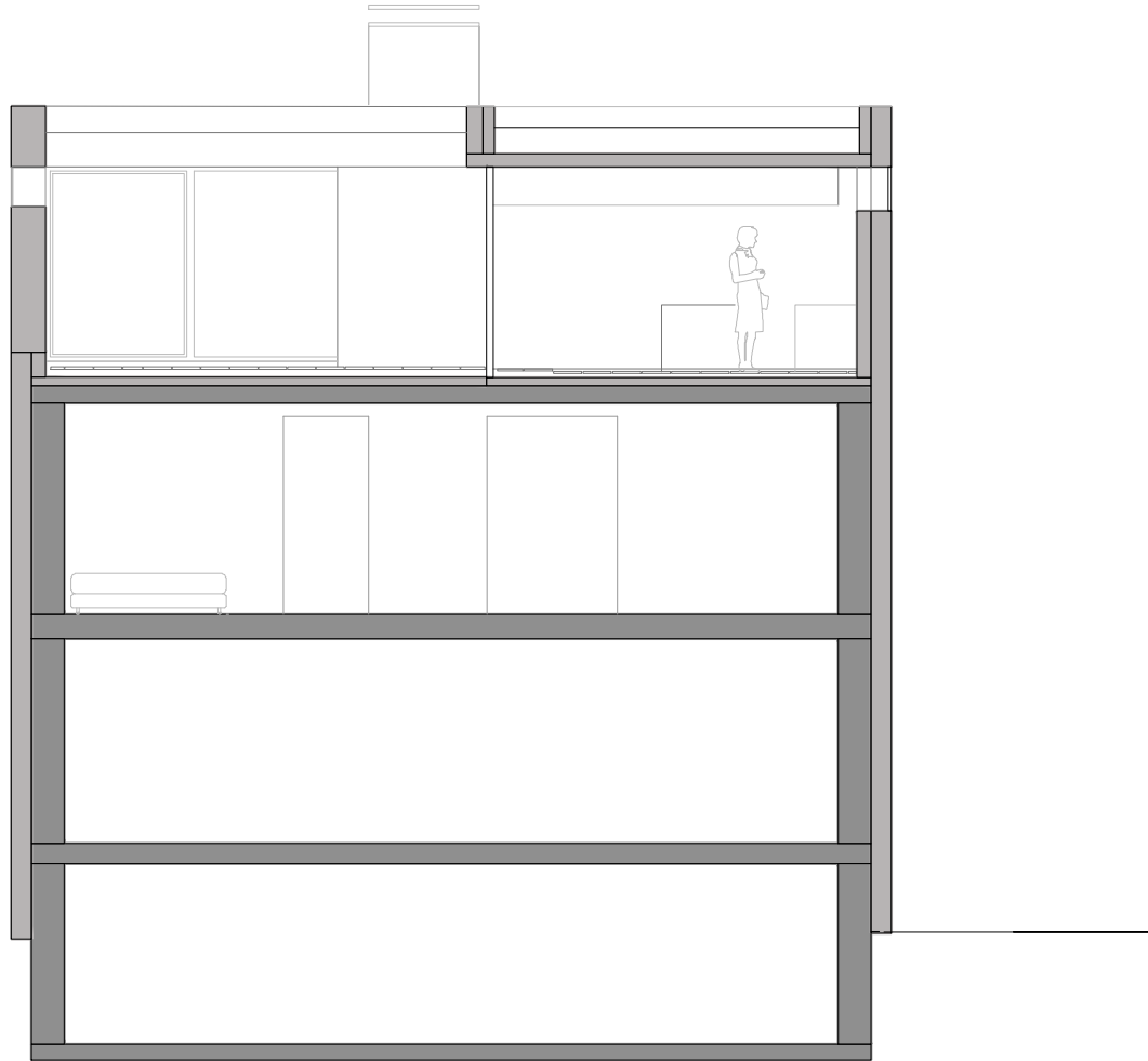
QUERSCHNITT
