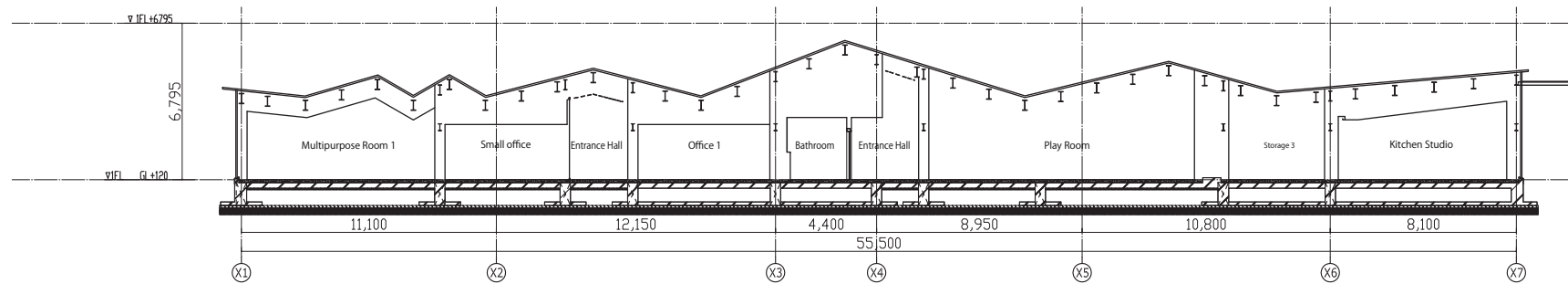
BB' section 1:300
