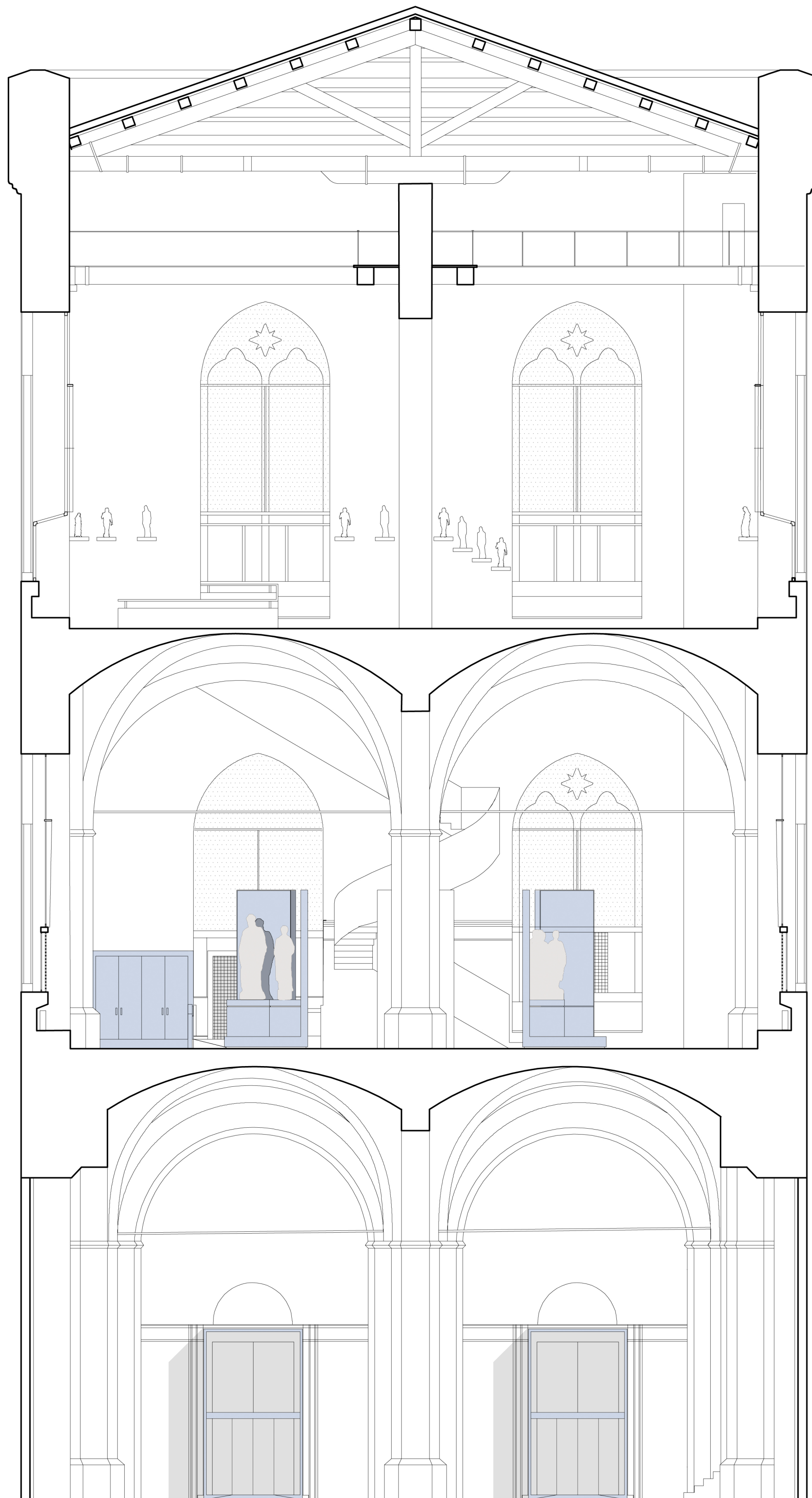
Sezione BB'
