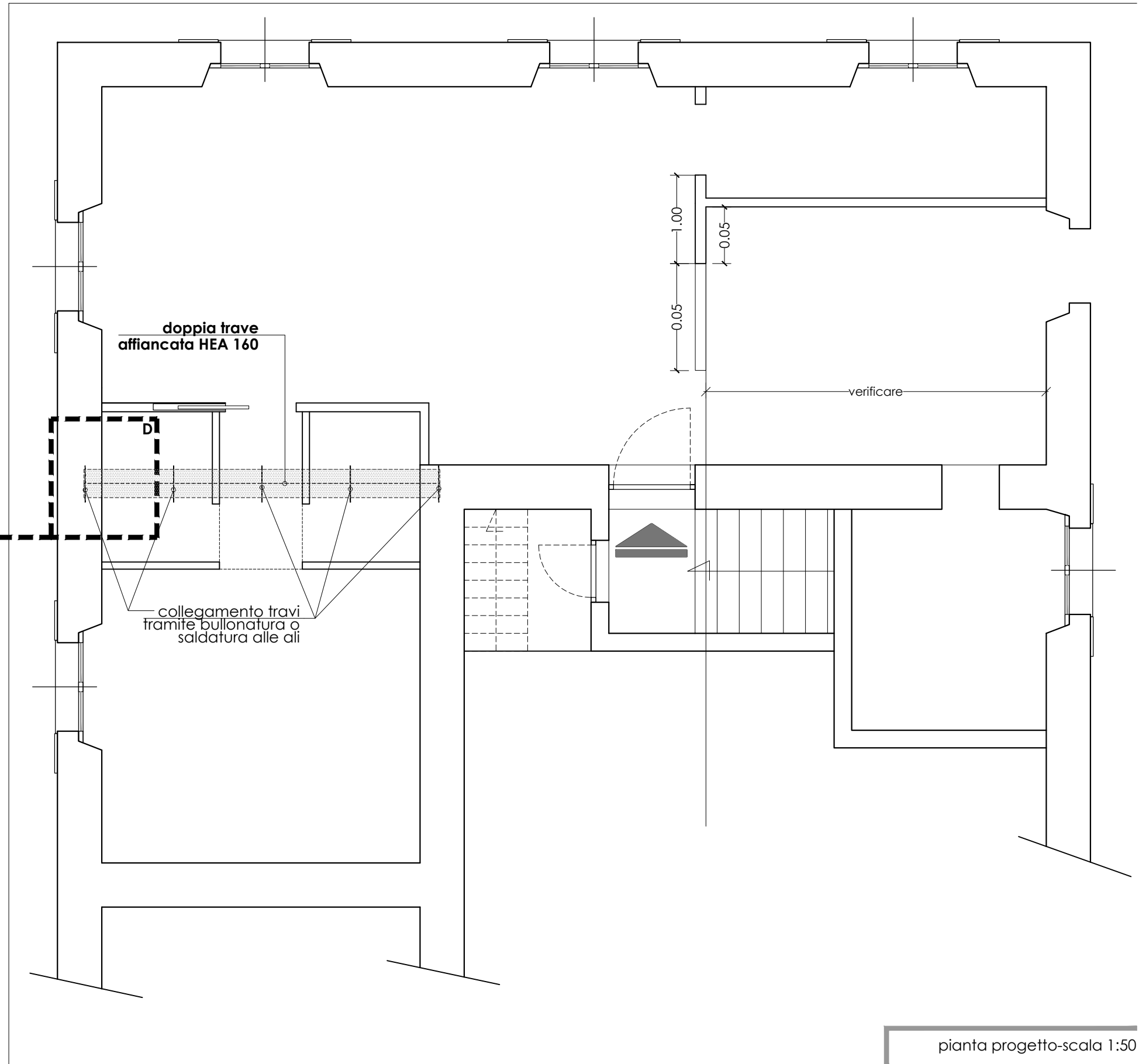
D - dettaglio architravatura scala 1:5
