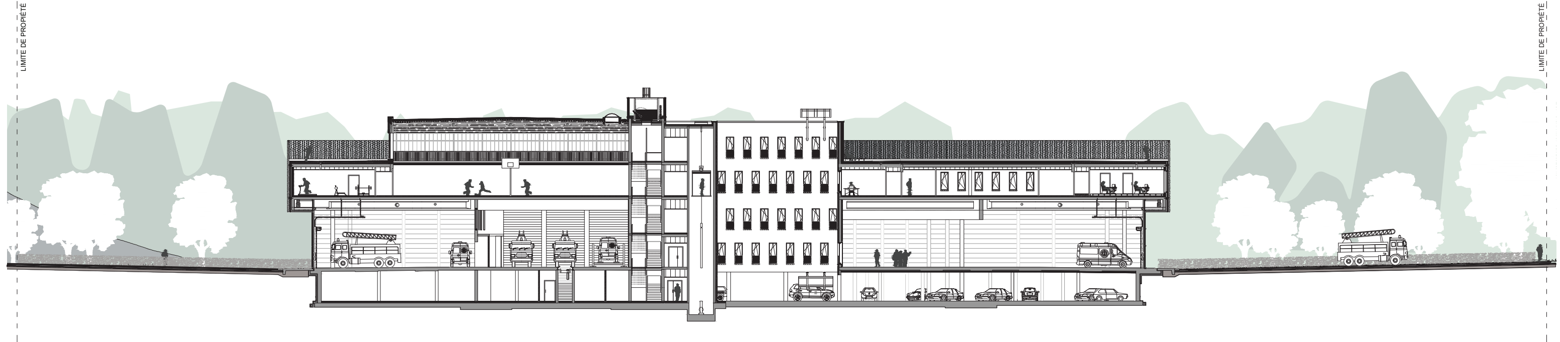
COUPE EE'
