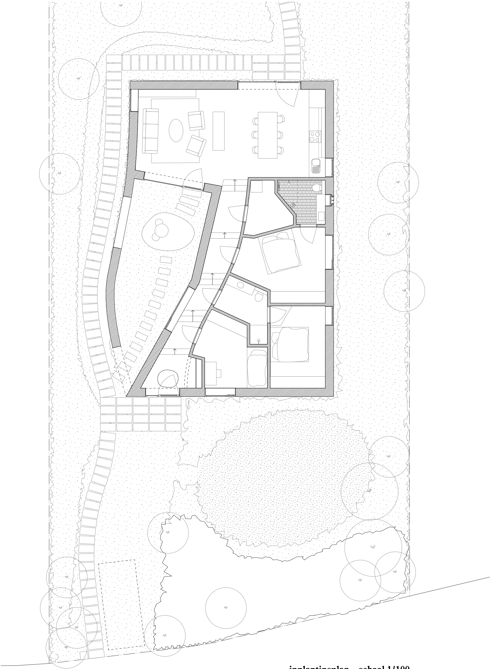
inplantinsplan - schaal 1/100
