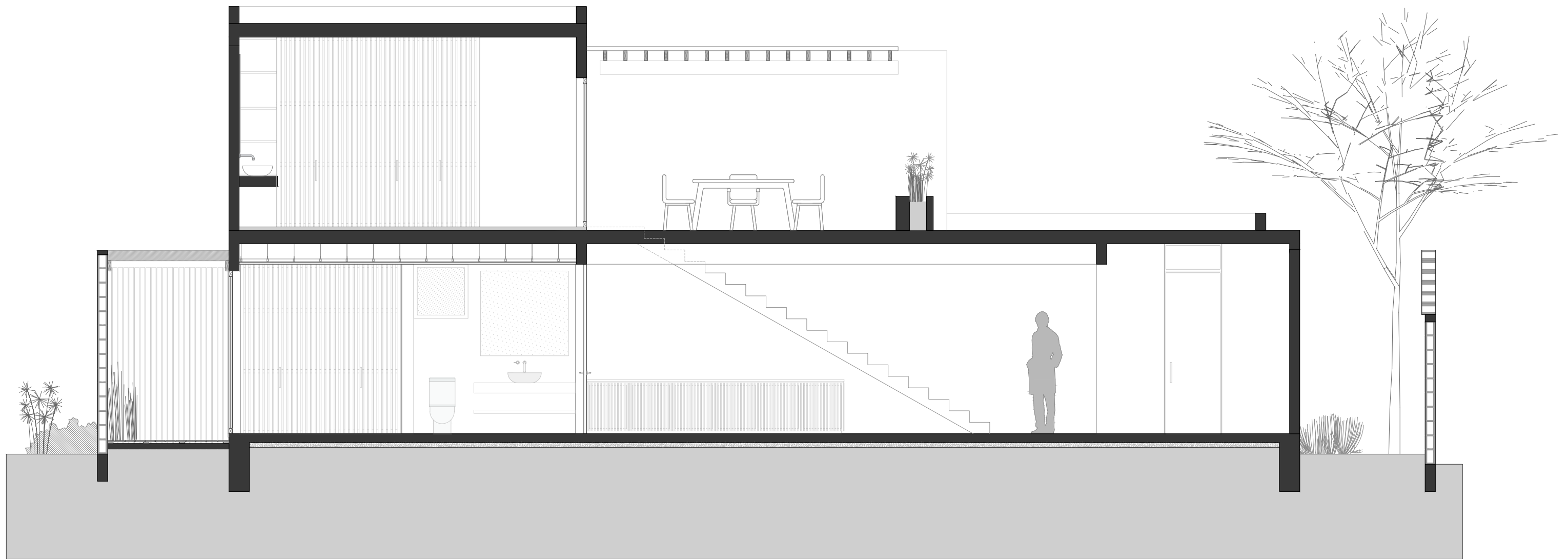
Villa 03 | Corte A-A'
