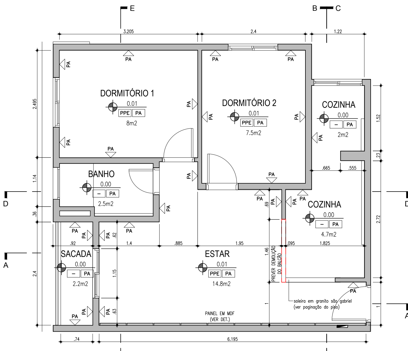
PLANTA Escala 1:50
