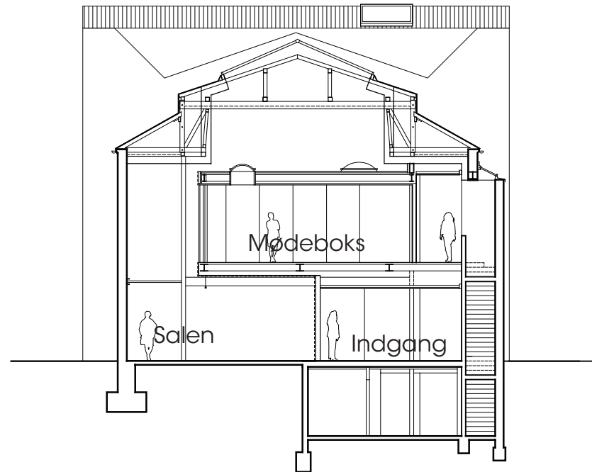
snit C-C 1:200
