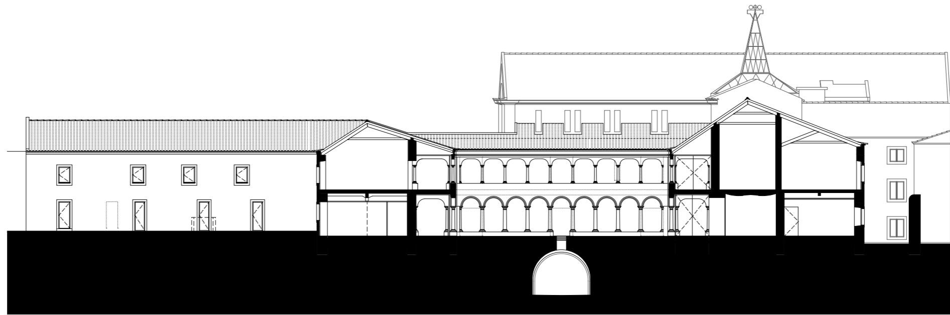
corte 1-1'. section 1-1'
