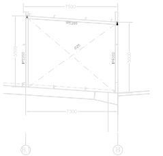
CASETÓN PÓRTICO TRANSVERSAL 17 y 18
