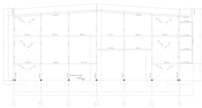
PÓRTICO TRANSVERSAL 1
