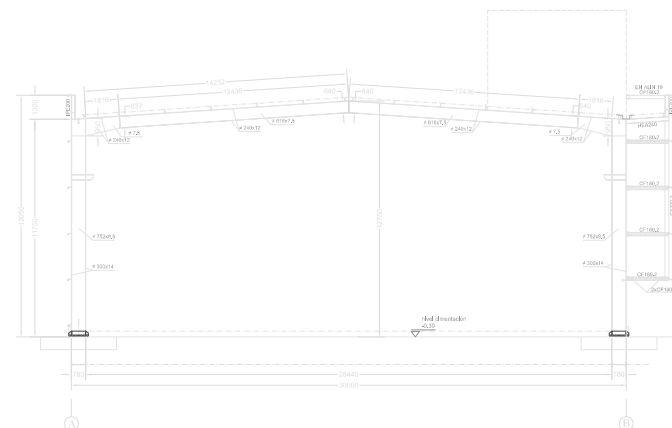
PÓRTICO TRANSVERSAL 16, 17 y 19
