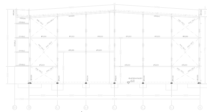
PÓRTICO TRANSVERSAL 20
