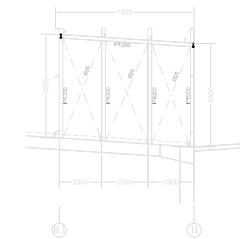
CASETÓN PÓRTICO TRANSVERSAL 16 y 19
