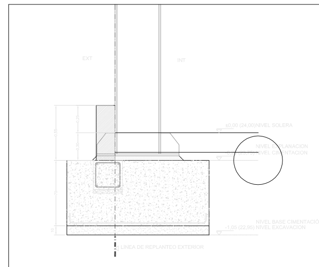
DETALLE CONSTRUCTIVO
