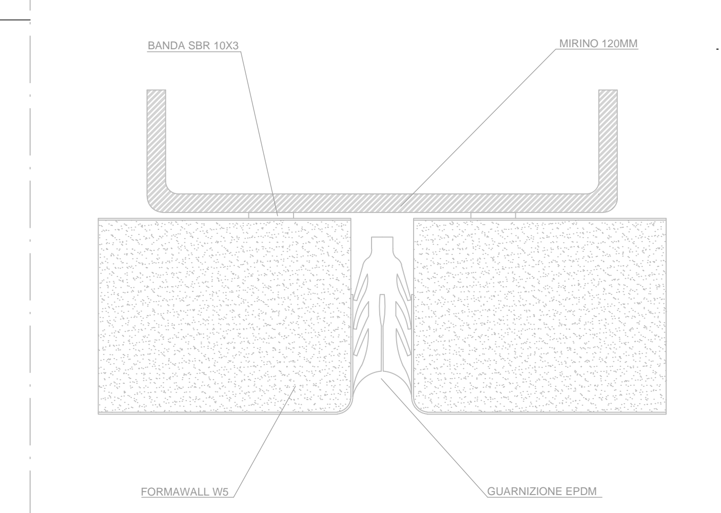
SEZIONE A-A'
