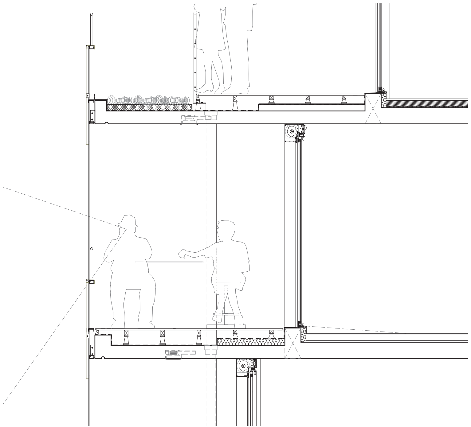
Détail sur balcons / terrasses - retrait supérieur
