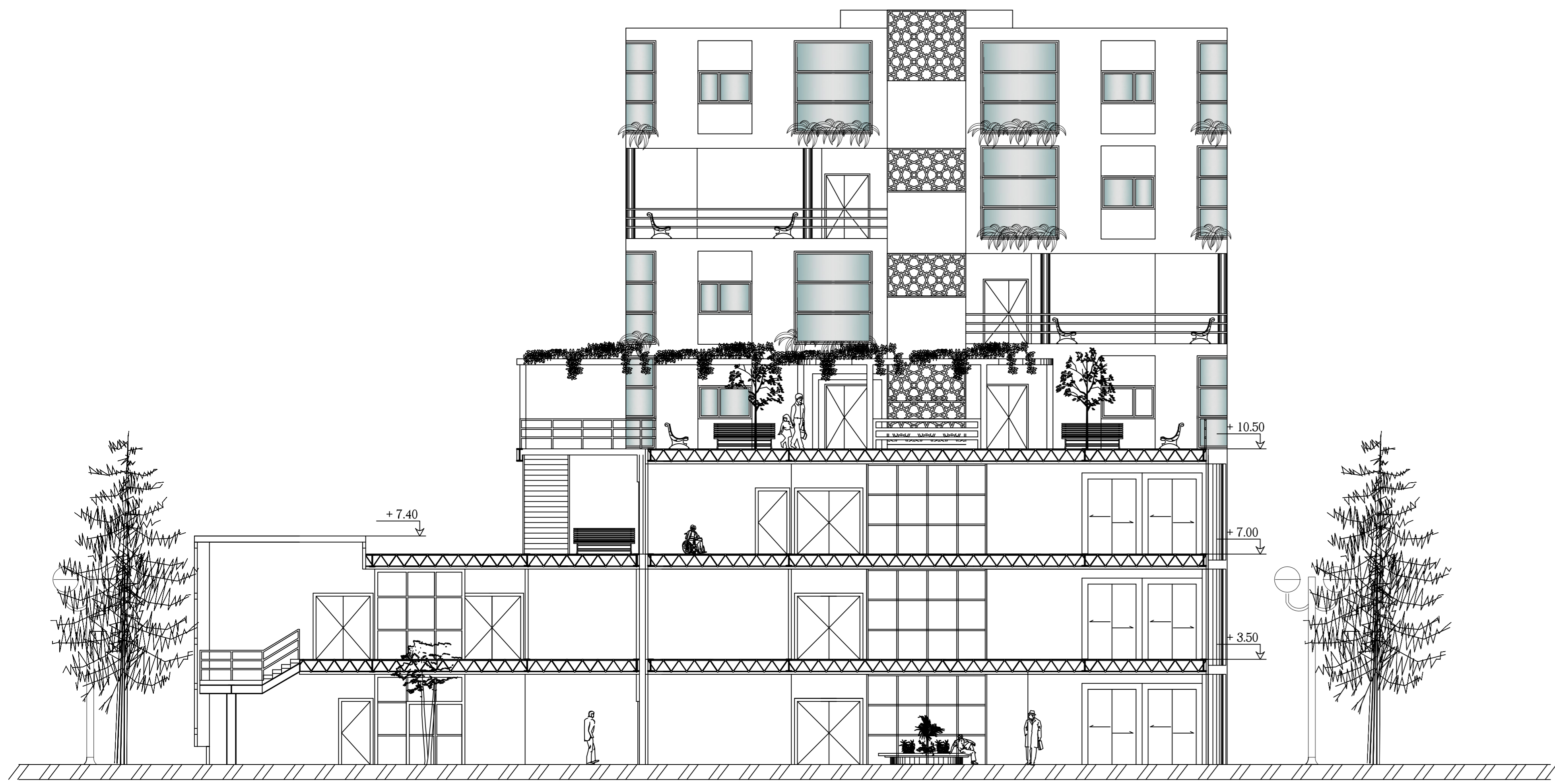
Coupe-AA
