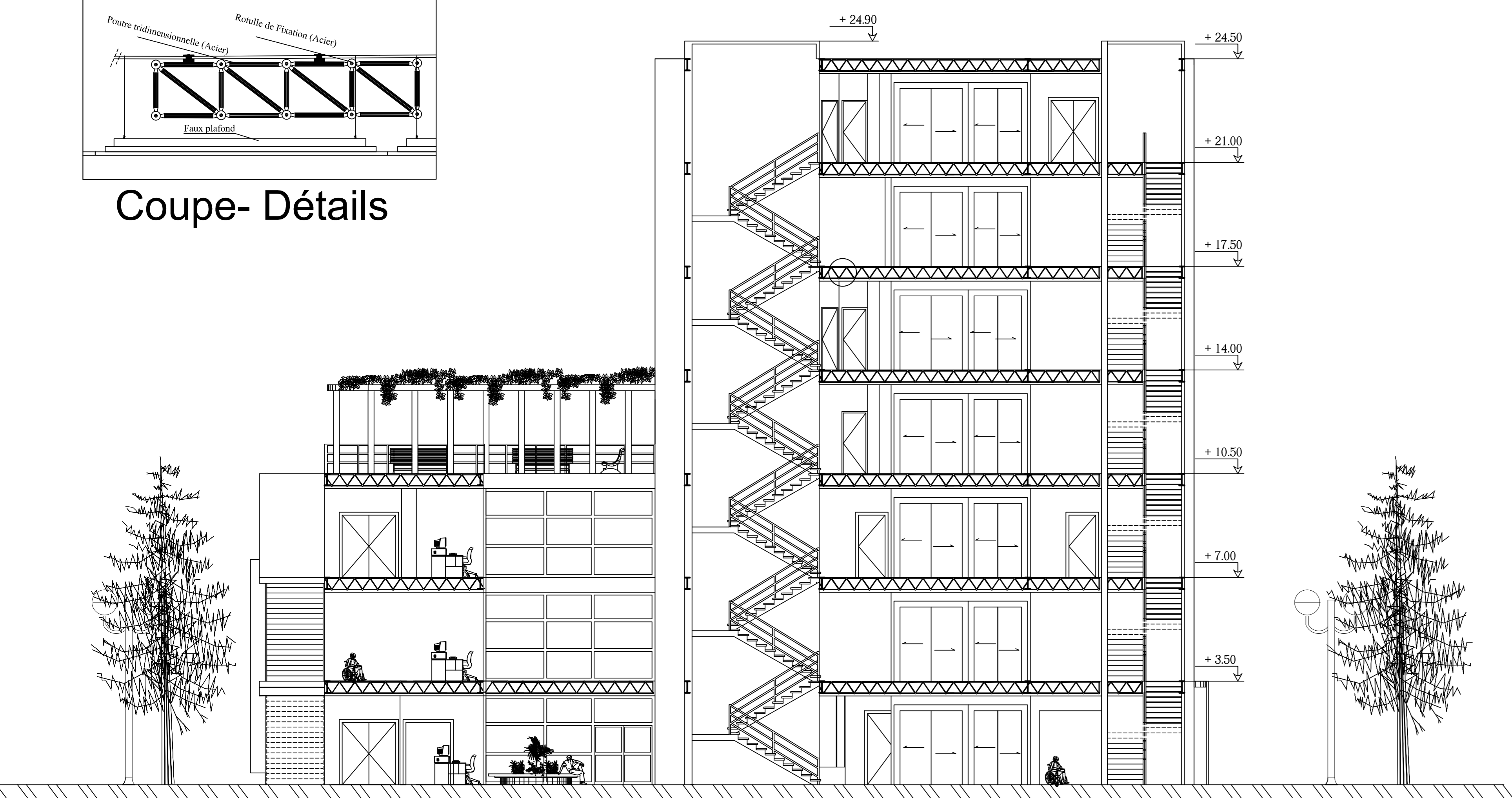
Coupe- BB
