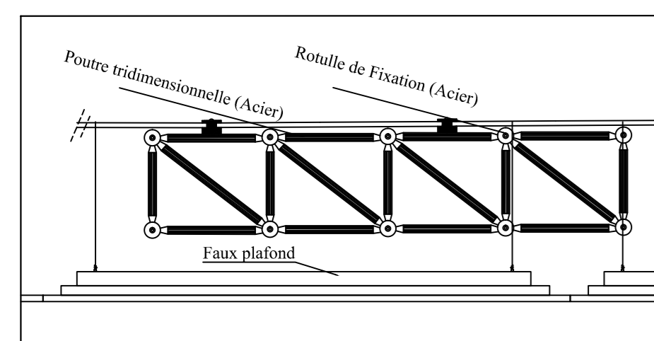
Coupe- Détails
