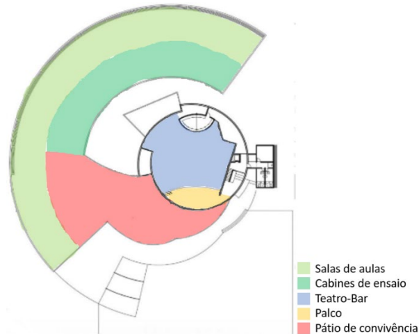
Figura 47: Planta baixa – Térreo.
