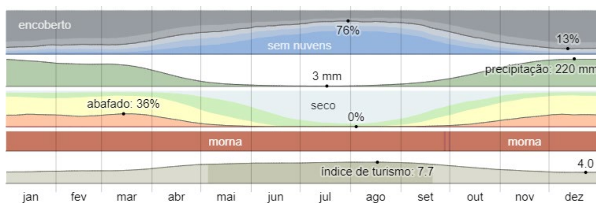
Figura 76: Imagem figurativa do clima do Distrito Federal
