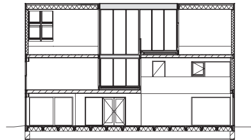
Doorsnede A-A'
