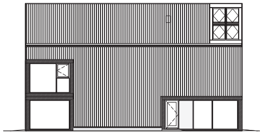
Straatgevel
