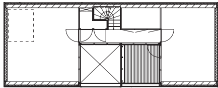
2e verdieping
