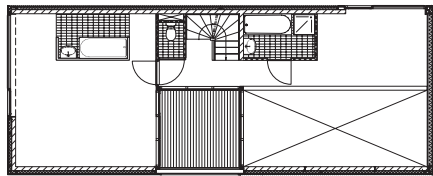
1e verdieping
