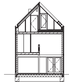
Doorsnede B-B'
