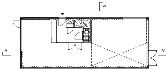
Begane grond
