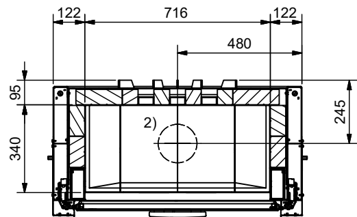
Grundriss Feuerstelle / Coupe sur foyer Sezione al piano fuoco / Layout fireplace
