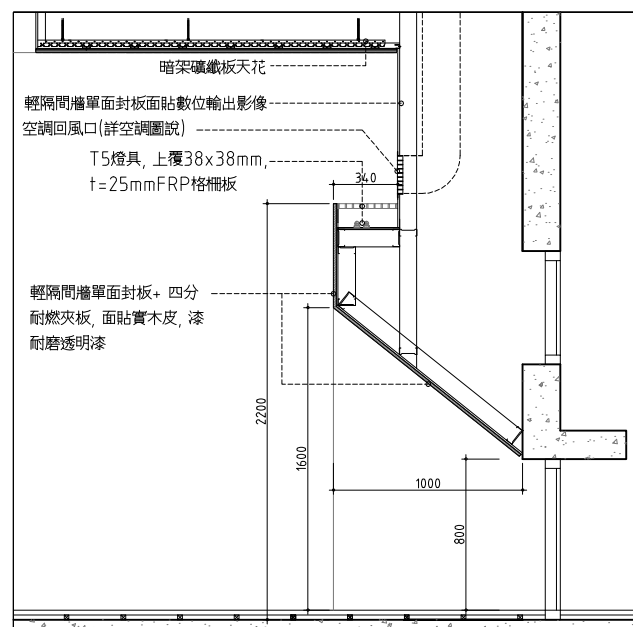
11 五層壁櫃 TYPE B 剖面詳圖 SCALE: 1/20 UNIT: mm
