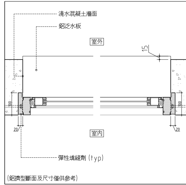
07 開口標準詳圖(側面平面) SCALE: 1/5 UNIT: mm
