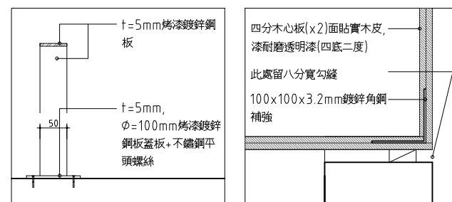
06 樓梯下金屬護欄 剖面詳圖 SCALE: 1/5 UNIT: mm
