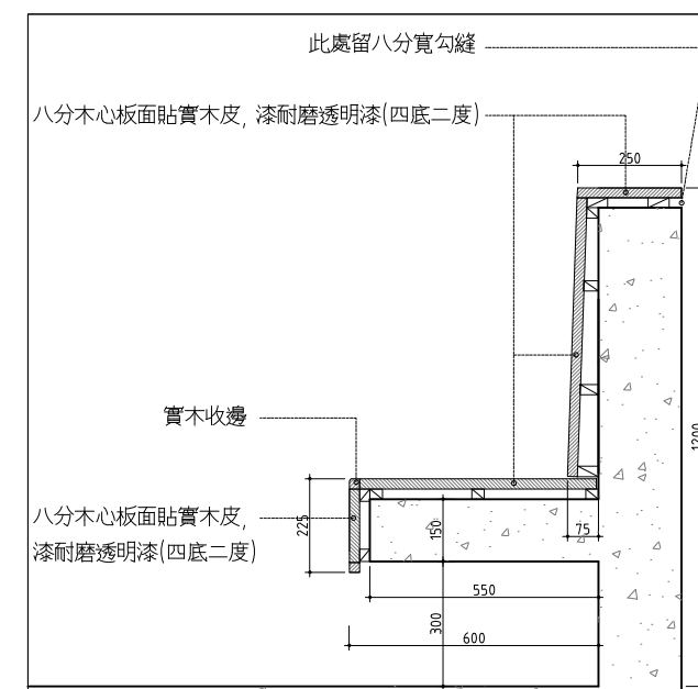
12 2/3/4F立式檢索台暨帶狀座椅 剖面詳圖(座位區) SCALE: 1/10 UNIT: mm
