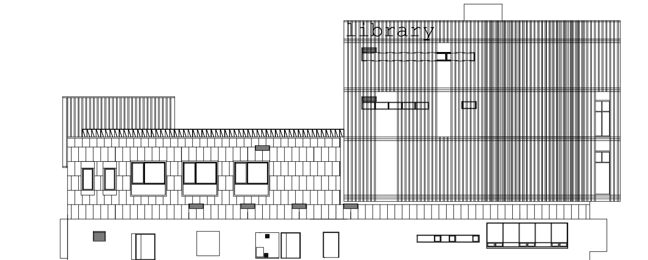
北向立面圖 unit:m | 0 | 2 | 5 | 10
