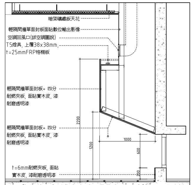
08 五層壁櫃 TYPE B 剖面詳圖 SCALE: 1/20 UNIT: mm
