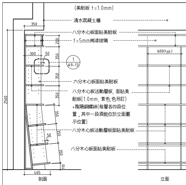
05 六層壁櫃詳圖 SCALE: 1/20 UNIT: mm
