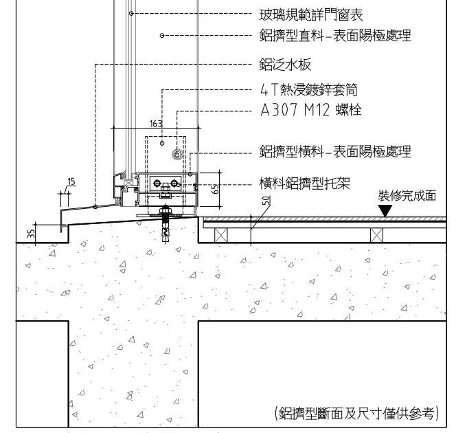
12 玻璃帷幕窗剖面詳圖(下部) SCALE: 1/5 UNIT: mm
