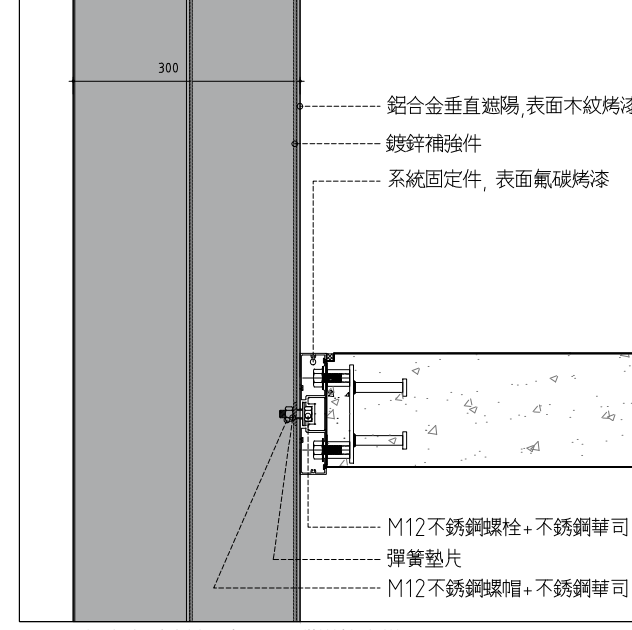
11 鋁合金垂直遮陽板及RC貓道接合詳圖 SCALE: 1/5 UNIT: mm
