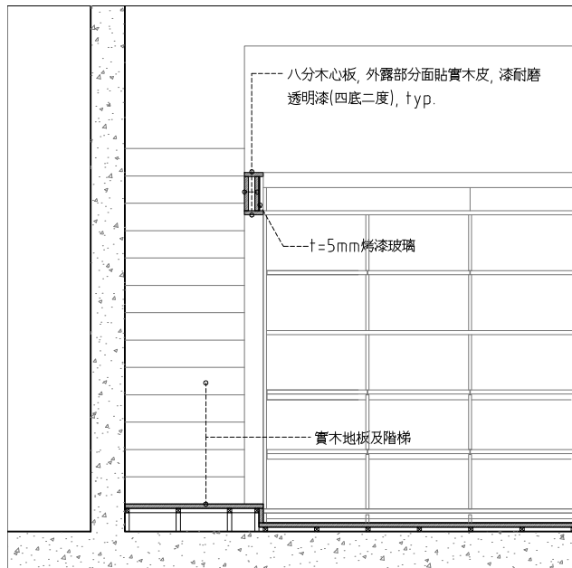
01 樹屋剖面詳圖 SCALE: 1/20 UNIT: mm
