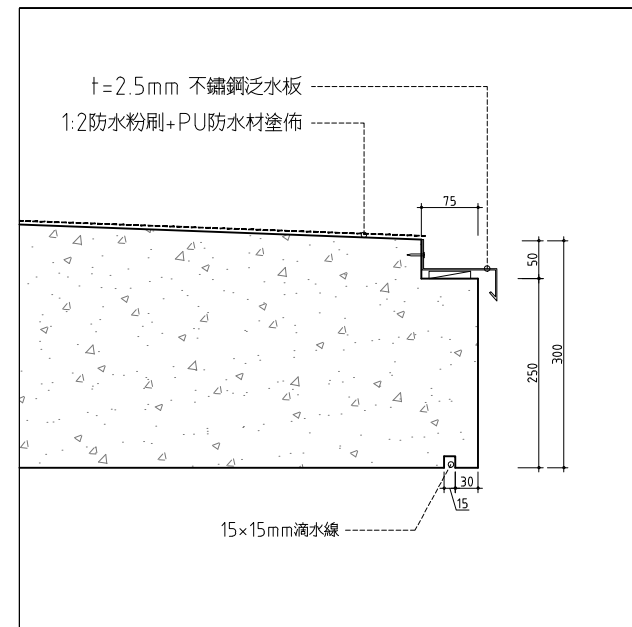
03 RC雨底邊緣詳圖 SCALE: 1/5 UNIT: mm
