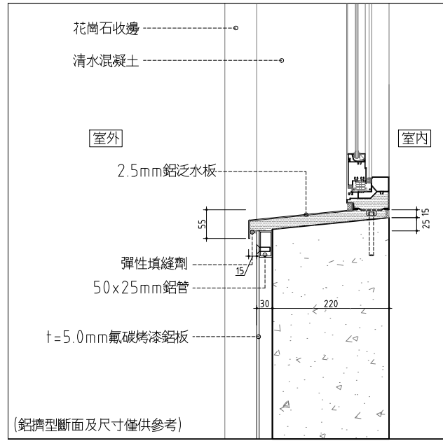
05 W8窗詳圖(下部剖面) SCALE: 1/5 UNIT: mm
