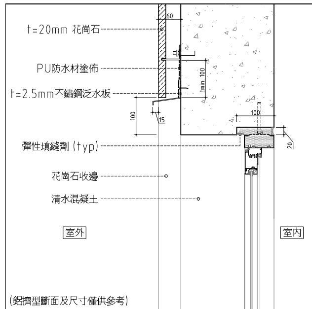
01 外掛石板+RC牆界面詳圖/W8窗詳圖(上部剖面) SCALE: 1/5 UNIT: mm
