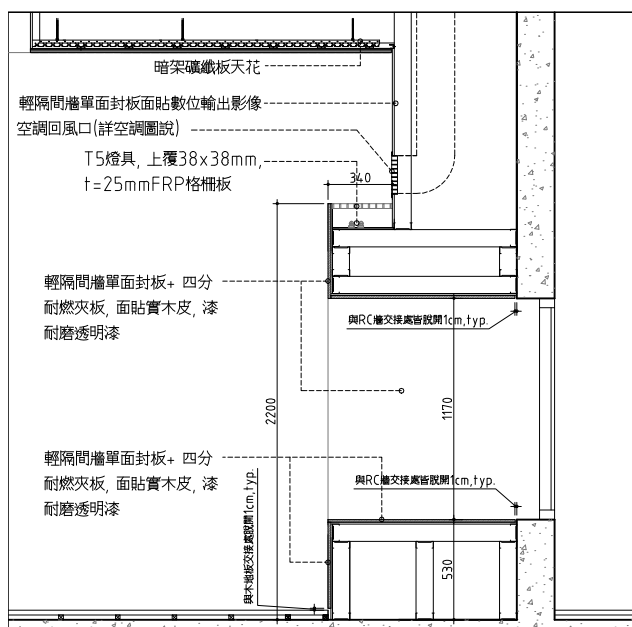
09 五層壁櫃 TYPE B 剖面詳圖 SCALE: 1/20 UNIT: mm
