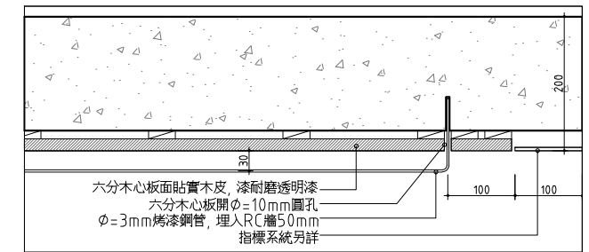
03 新書展示台 書架詳圖 SCALE: 1/5 UNIT: mm
