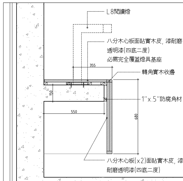
04 靠窗座椅 剖面詳圖(桌面區) SCALE: 1/10 UNIT: mm
