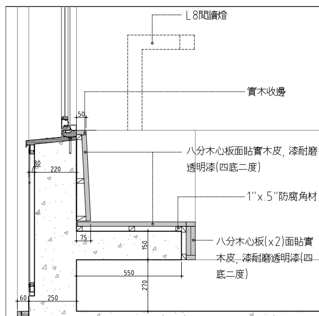
10 靠窗座椅 剖面詳圖(座位區) SCALE: 1/10 UNIT: mm
