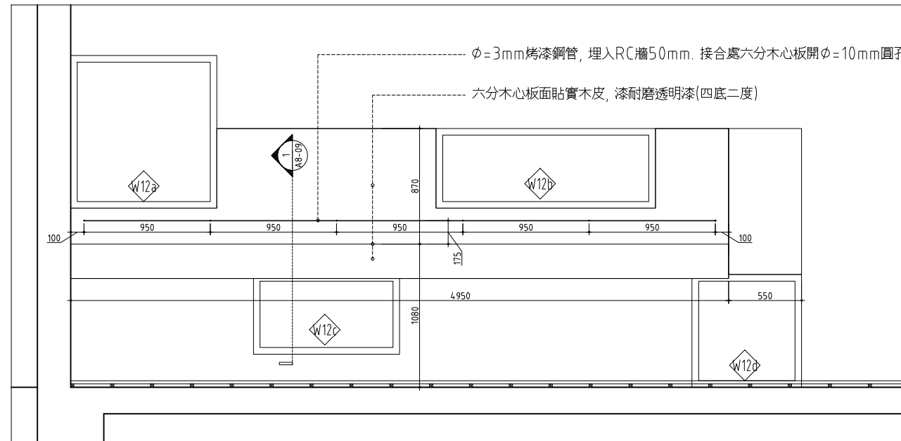
02 新書展示台 立面詳圖 SCALE: 1/20 UNIT: mm
