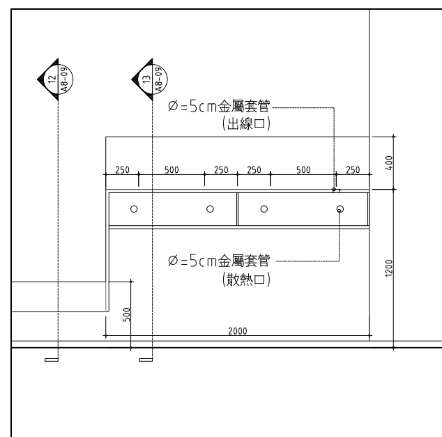
11 3/4F立式檢索台暨帶狀座椅 立面詳圖 SCALE: 1/20 UNIT: mm
