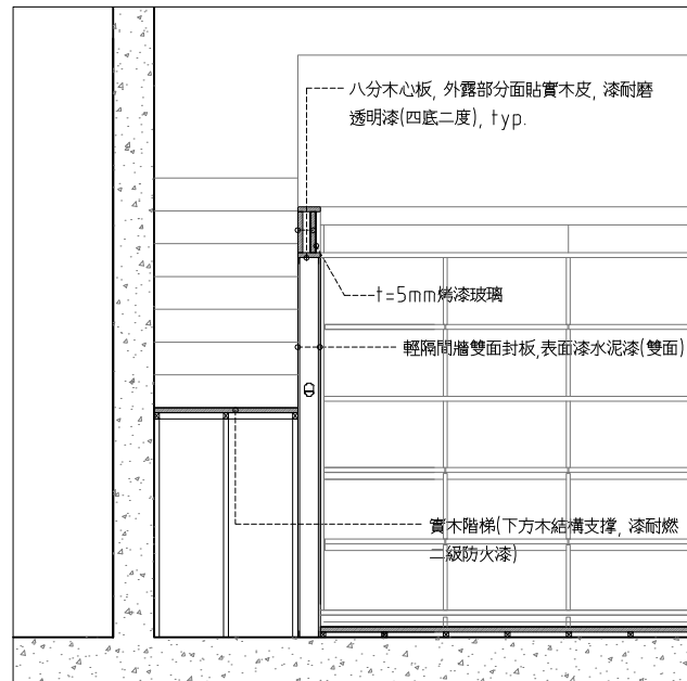
02 樹屋剖面詳圖 SCALE: 1/20 UNIT: mm
