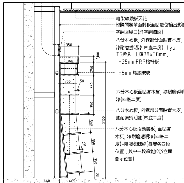
06 五層壁櫃 TYPE A 詳圖 SCALE: 1/20 UNIT: mm
