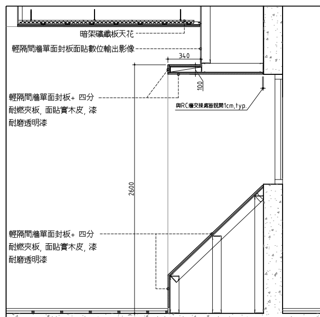
10 五層壁櫃 TYPE B 剖面詳圖 SCALE: 1/20 UNIT: mm
