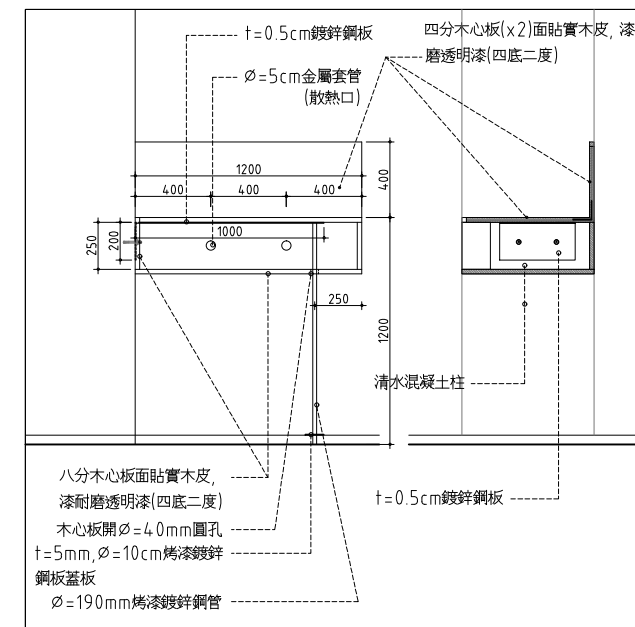
07 2/3/4F立式檢索台詳圖 SCALE: 1/5 UNIT: mm
