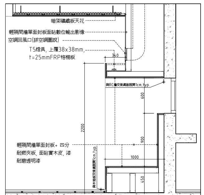
12 五層壁櫃 TYPE B 剖面詳圖 SCALE: 1/20 UNIT: mm
