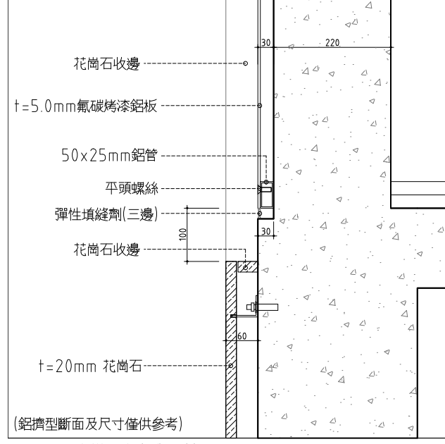
09 W8窗詳圖(鋁板與石材界面) SCALE: 1/5 UNIT: mm
