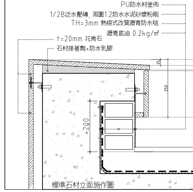
10 屋頂女兒牆詳圖 SCALE: 1/5 UNIT: mm
