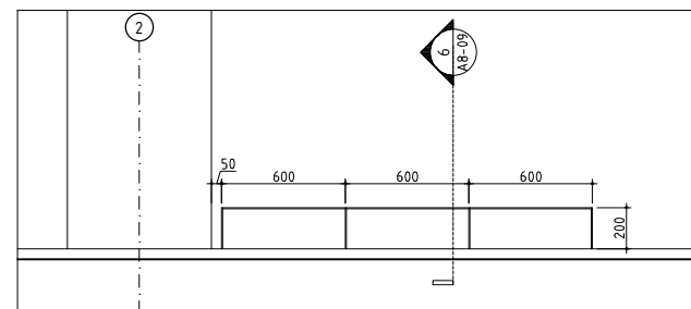
05 樓梯下金屬護欄 立面詳圖 SCALE: 1/20 UNIT: mm
