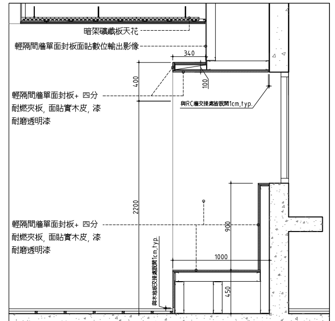
04 五層壁櫃 TYPE B 剖面詳圖 SCALE: 1/20 UNIT: mm
