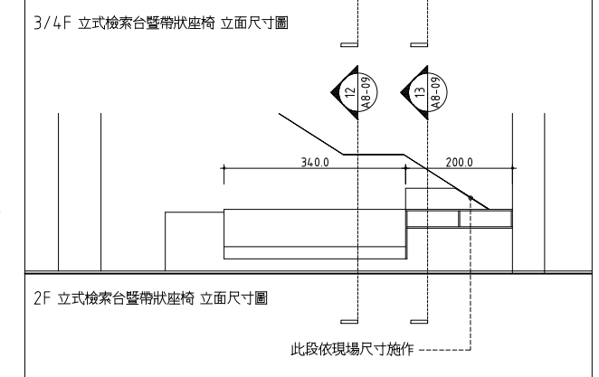
08 2F立式檢索架 詳圖 SCALE: 1/20 UNIT: mm
