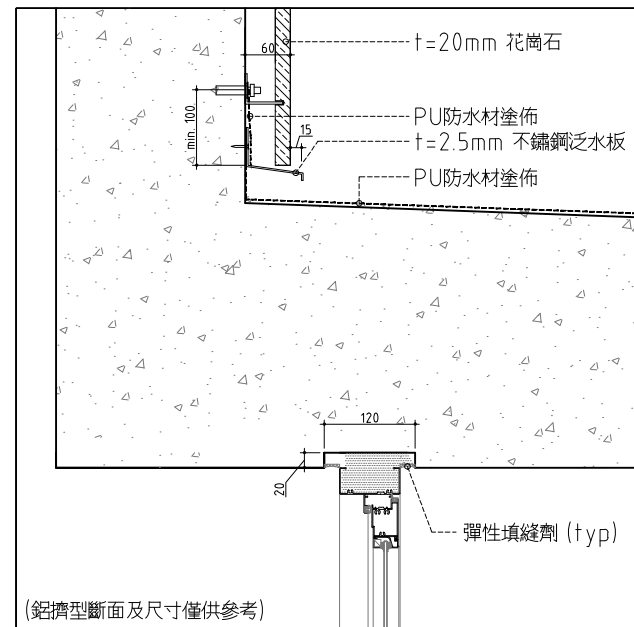
02 外掛石板+RC雨底界面詳圖/W7窗詳圖(上部剖面) SCALE: 1/5 UNIT: mm
