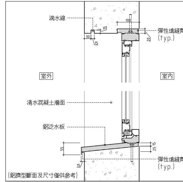
07 開口標準詳圖(剖面) SCALE: 1/5 UNIT: mm
