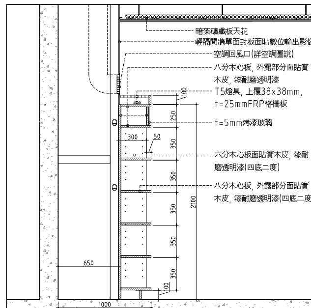
07 五層壁櫃 TYPE B 詳圖 SCALE: 1/20 UNIT: mm
