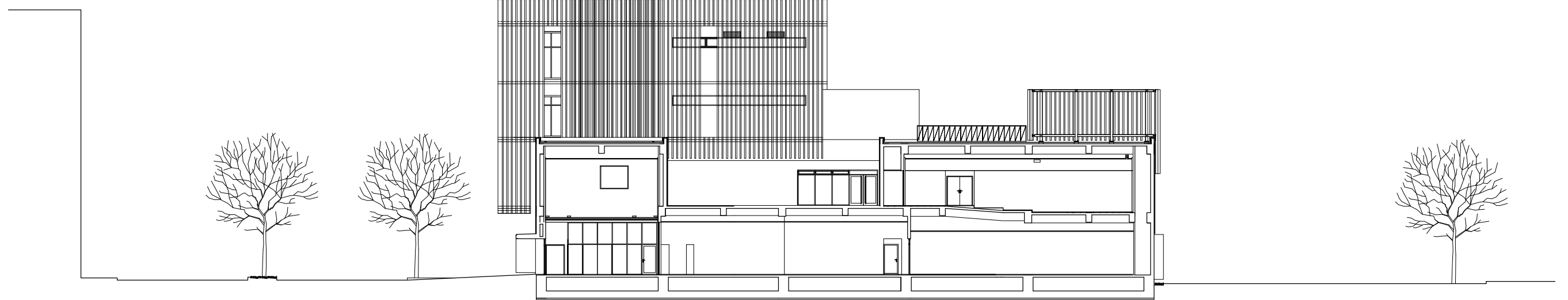
橫向剖面圖
