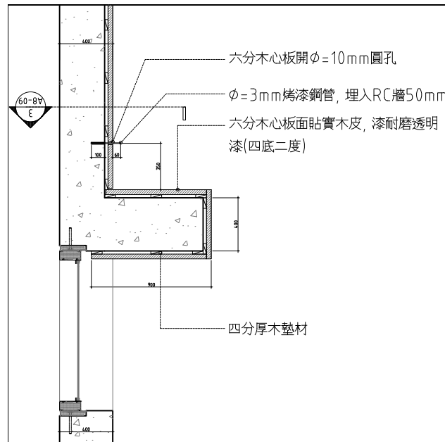
01 新書展示台 剖面詳圖 SCALE: 1/10 UNIT: mm
