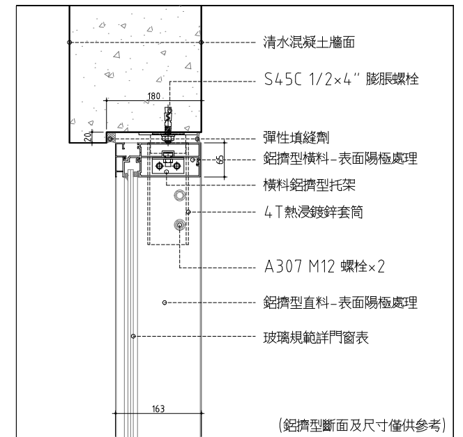
04 玻璃帷幕窗剖面詳圖(上部) SCALE: 1/5 UNIT: mm
