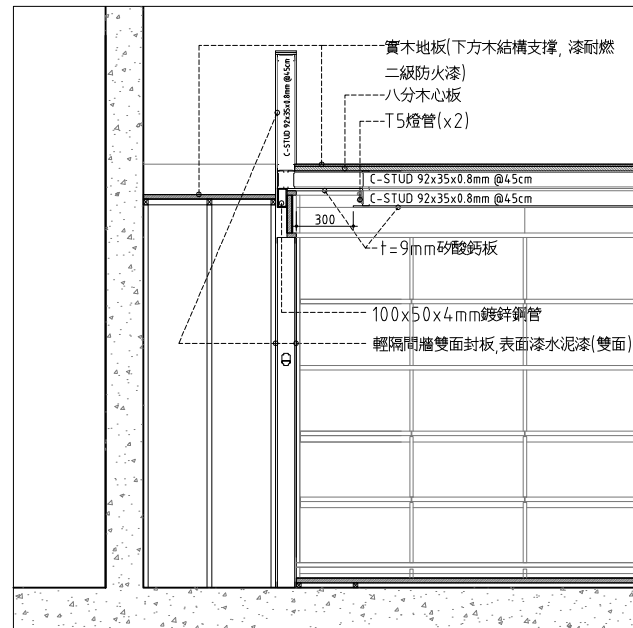
03 樹屋剖面詳圖 SCALE: 1/20 UNIT: mm
