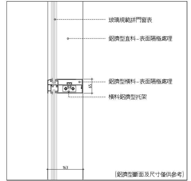
08 玻璃帷幕窗剖面詳圖(中段)開口標準詳圖(剖面) SCALE: 1/5 UNIT: mm
