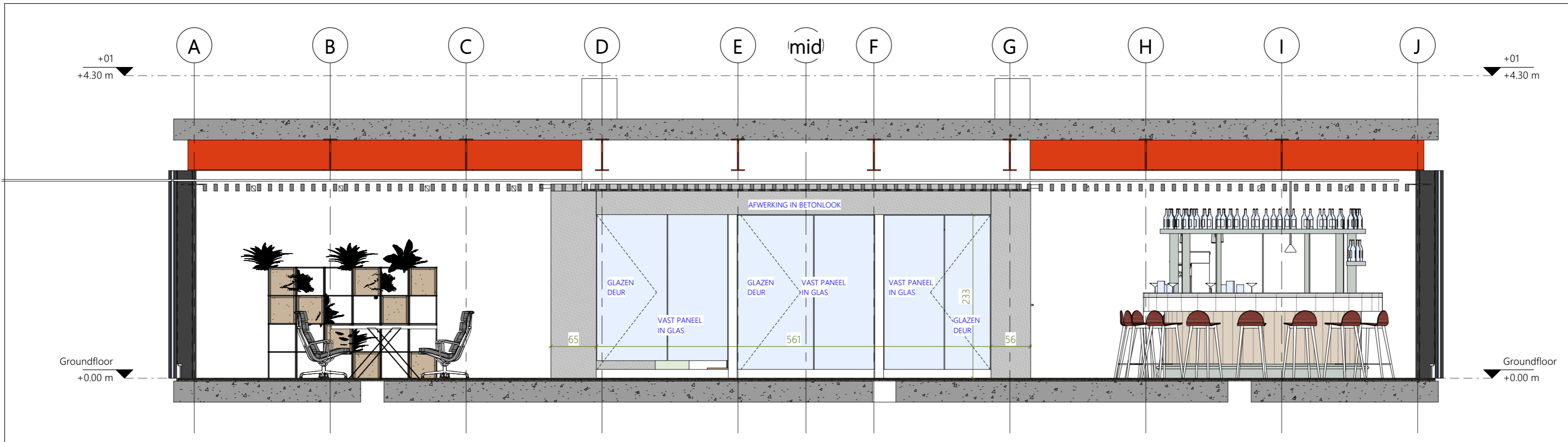
SNEDE CC (schaal: 1/50)
