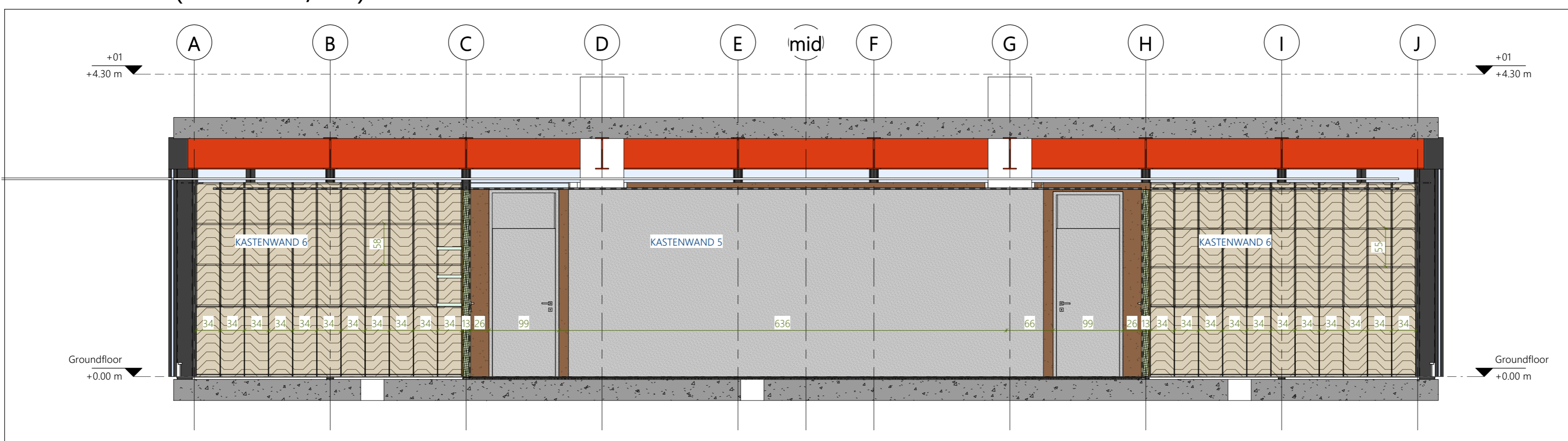
SNEDE EE (schaal: 1/50)
