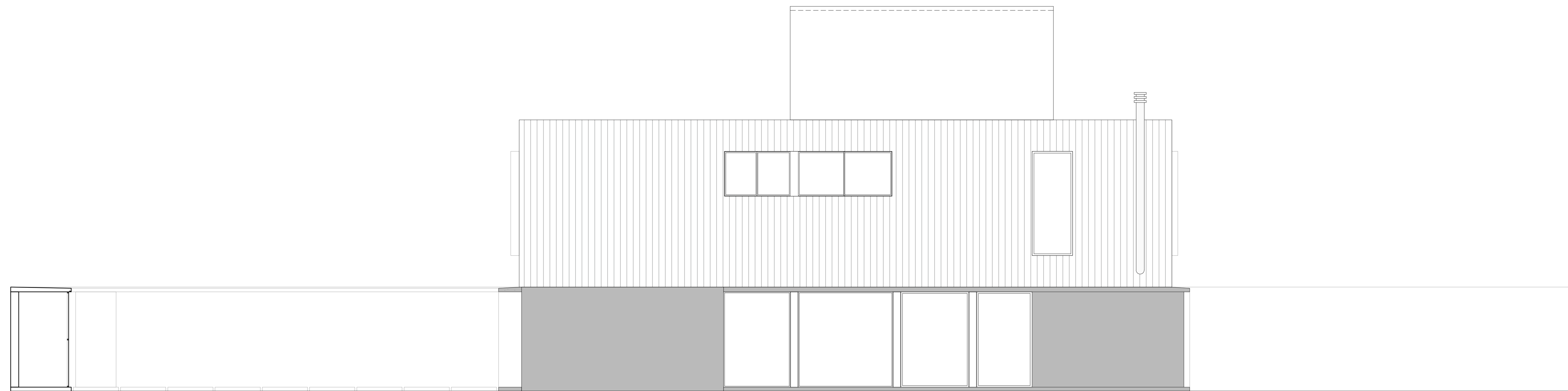
ELEVAÇÃO 3 - FACHADA LATERAL NORTE
