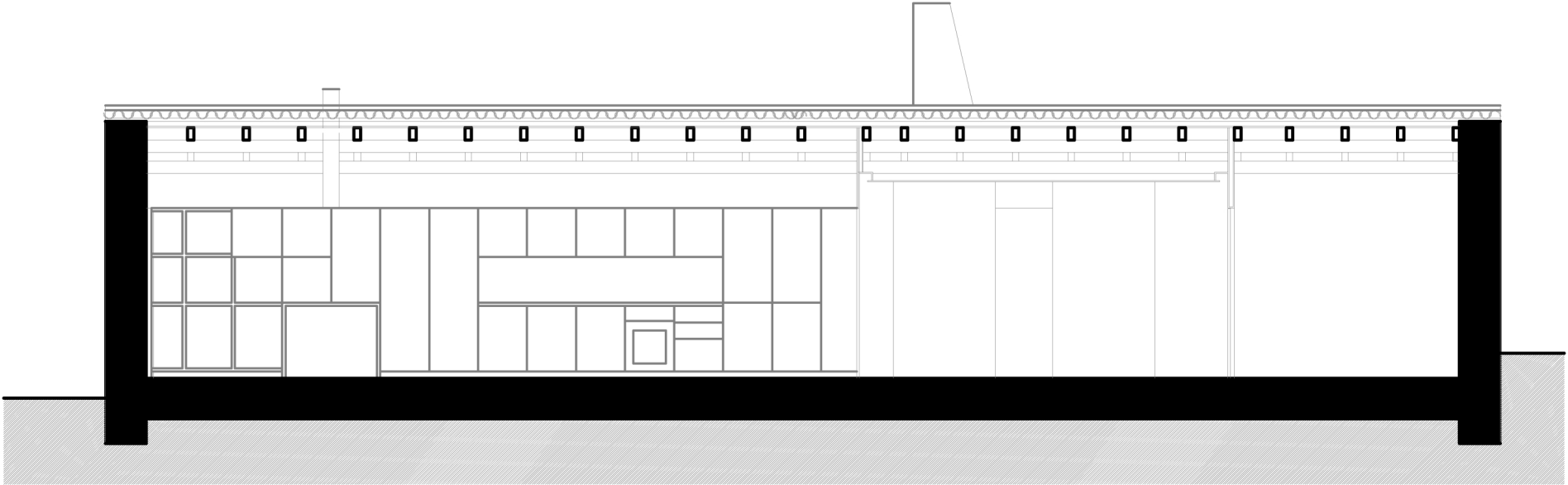
corte longitudinal_ long section 1:100
