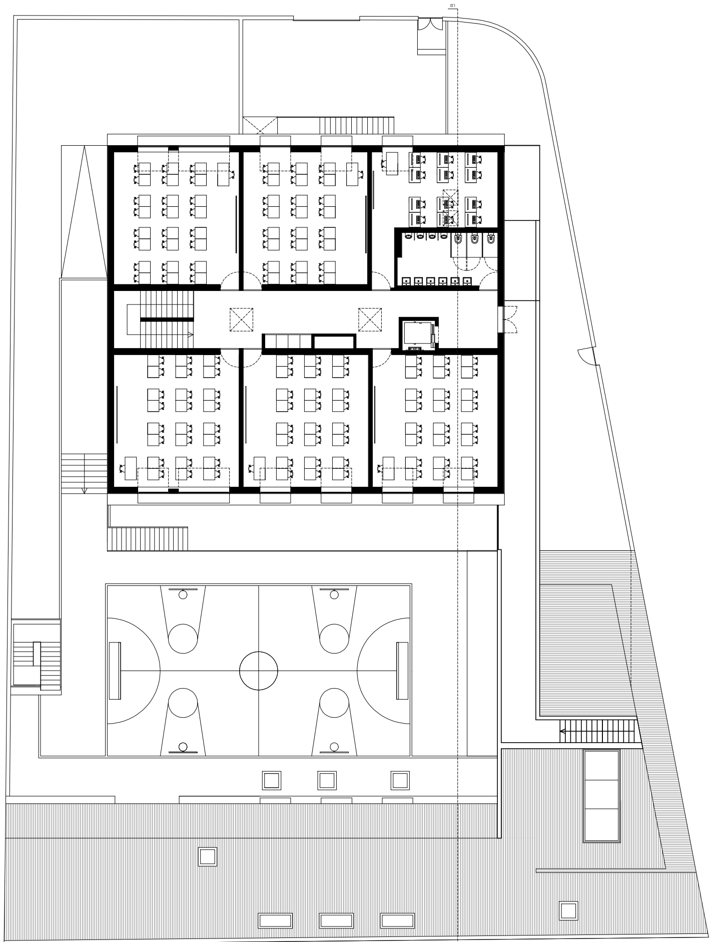
planta do piso 1
