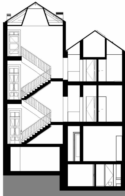
CORTE 02
