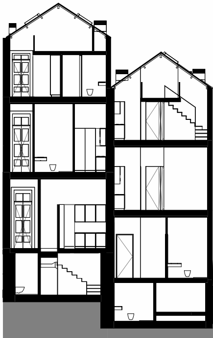
CORTE 01
