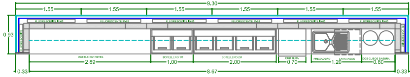
Planta de la barra del bar
