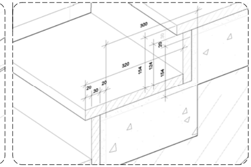
ქიბე 2 -ის საფეხურის დეტალი 4. მ. 1:5
