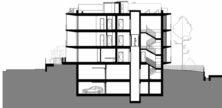
CORTE 01
