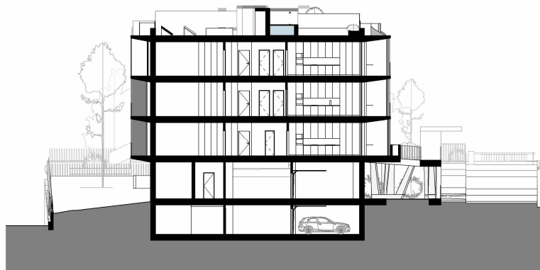
CORTE 02
