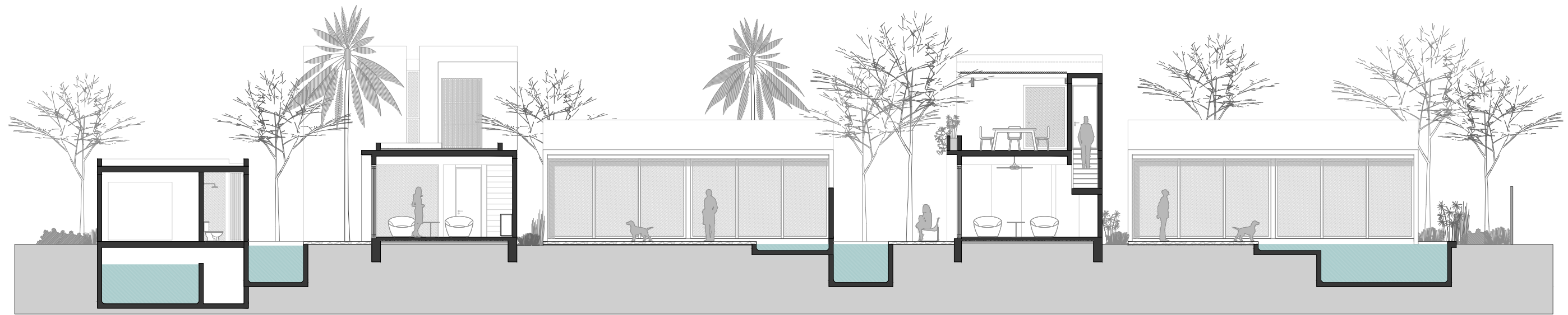
Corte Longitudinal Conjunto
