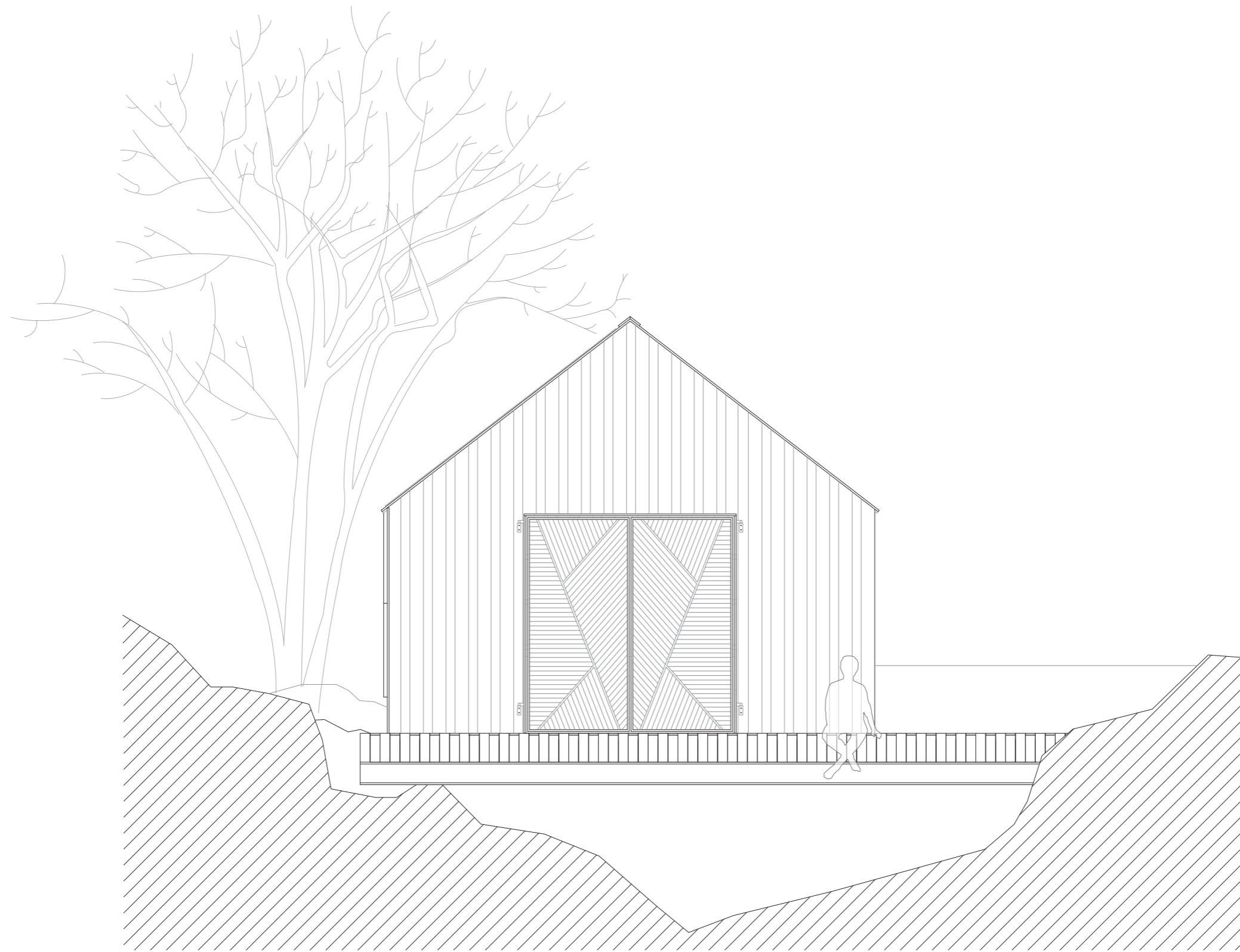
Fasade mot sjøen Målestokk 1:50
